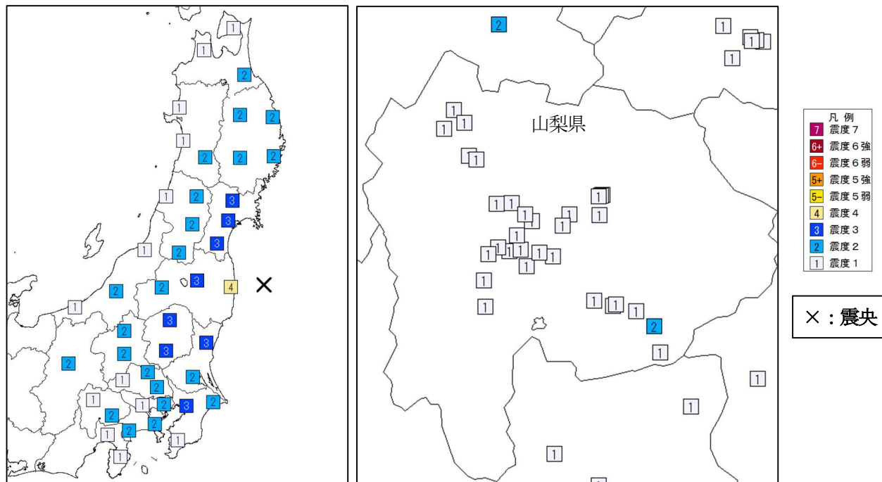
図1 震度分布図（5日00時21分 左図：地域別震度 右図：観測点別震度）
