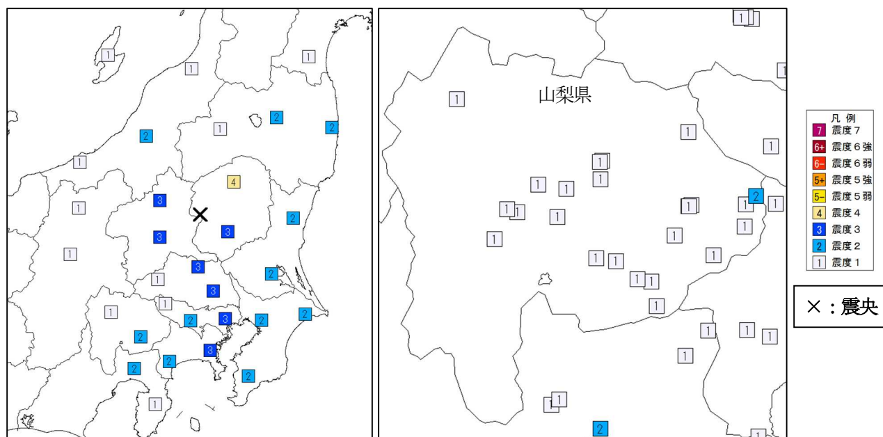
図2 震度分布図（26日12時04分 左図：地域別震度 右図：観測点別震度）
