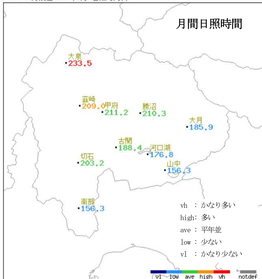
アメダス月別値 2023年3月 日照時間(h)
