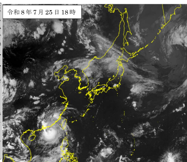
7月25日18時の地上天気図（左）と気象衛星赤外画像（右）
