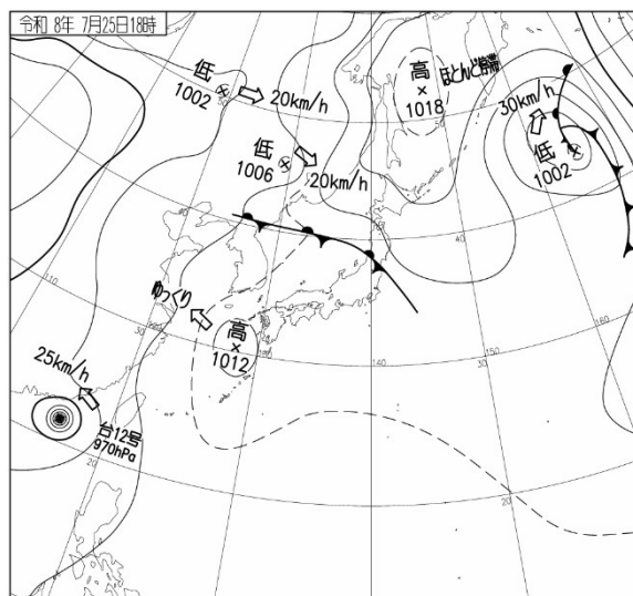
7月25日18時の地上天気図（左）と気象衛星赤外画像（右）
