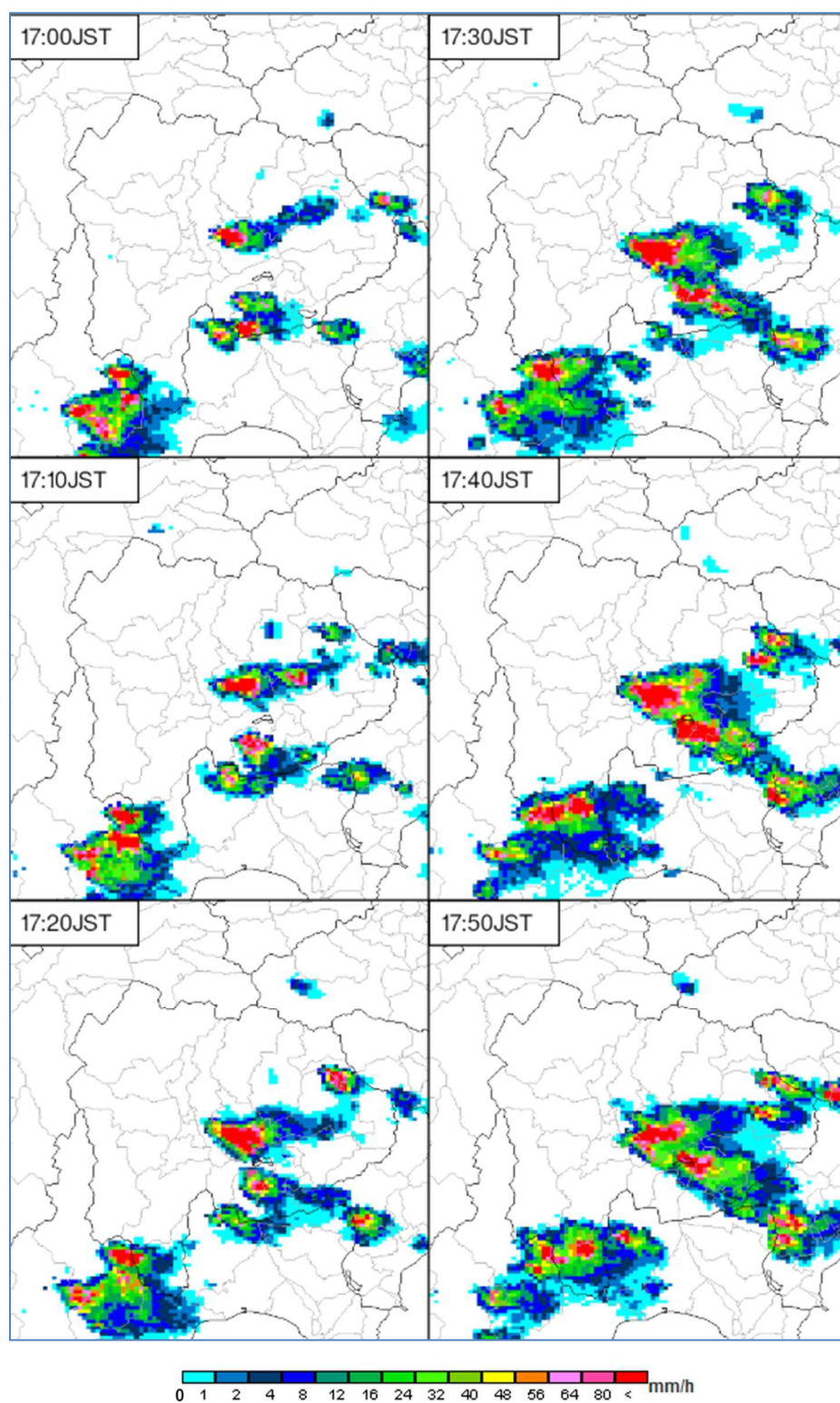
7月25日17時00分から10分毎のレーダー画像
