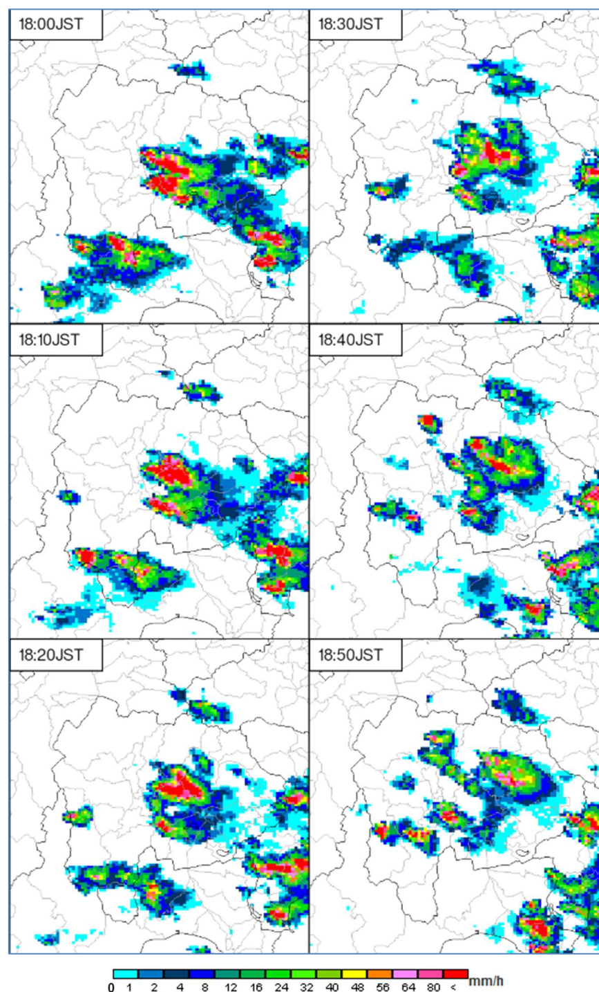
7月25日18時00分から10分毎のレーダー画像
