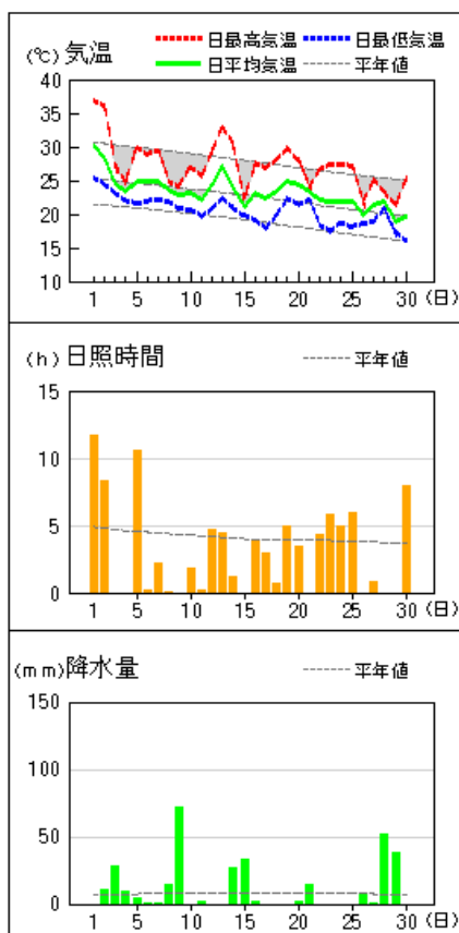
地上気象 気象経過図：2026年09月01日-2026年09月30日
