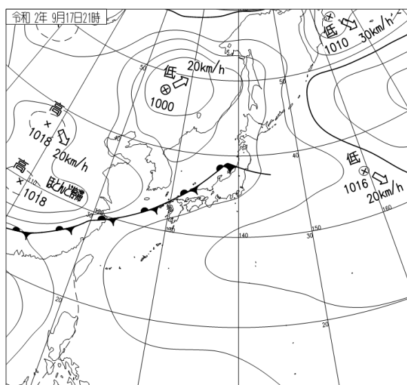
地上天気図（令和2年9月17日21時）
