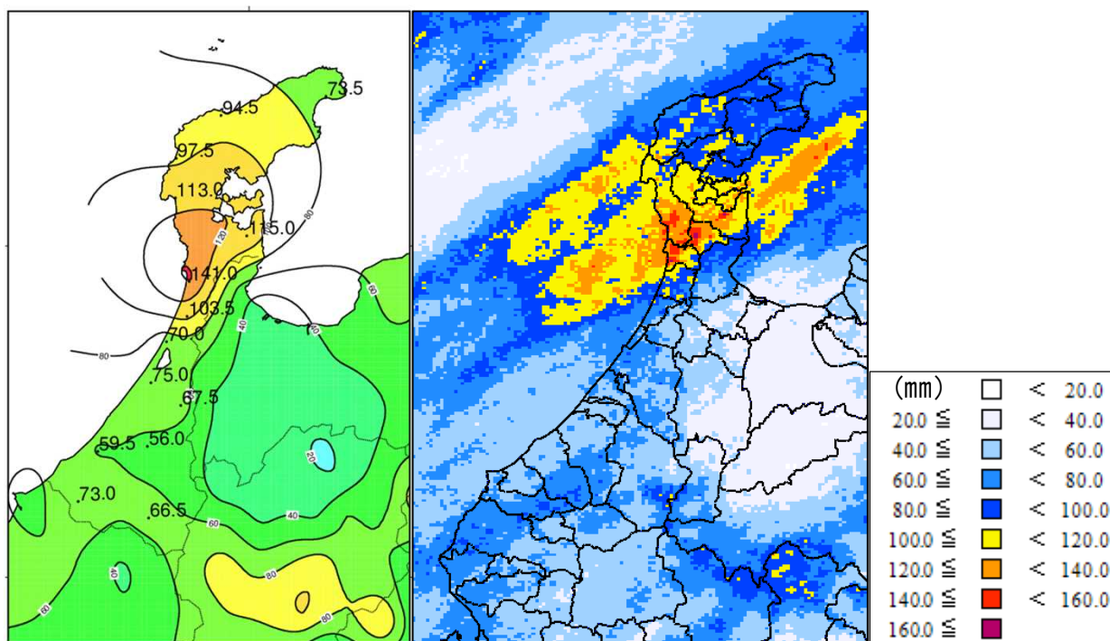
解析雨量の72時間積算値 （令和2年9月17日00時～19日24時）
