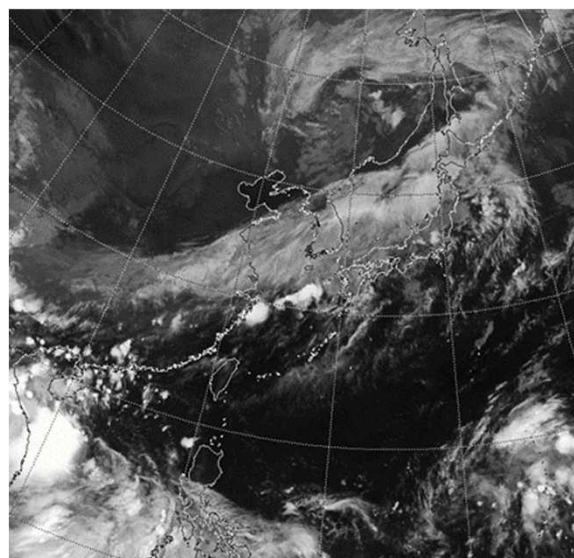
気象衛星赤外面像（令和2年9月17日21時）
