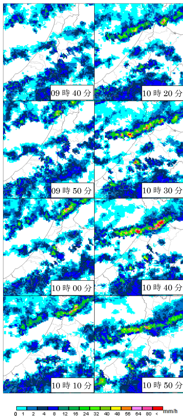
1月29日09時40分から10分毎のレーダー画像
