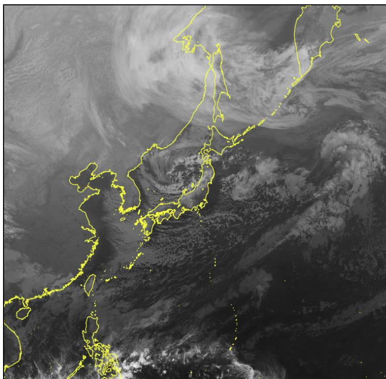
1 月 29 日 9 時 気象衛星赤外画像
