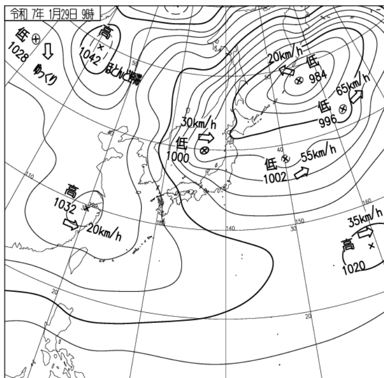
1 月 29 日 9 時 地上天気図
