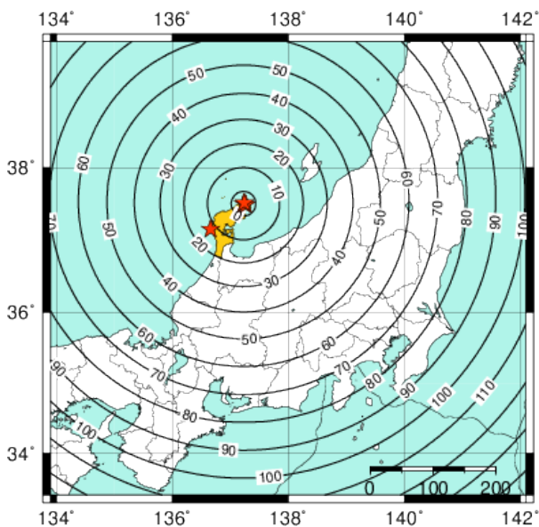
図6-1 警報第1報発表から主要動到達までの時間（秒）及び警報発表対象地域の分布図
