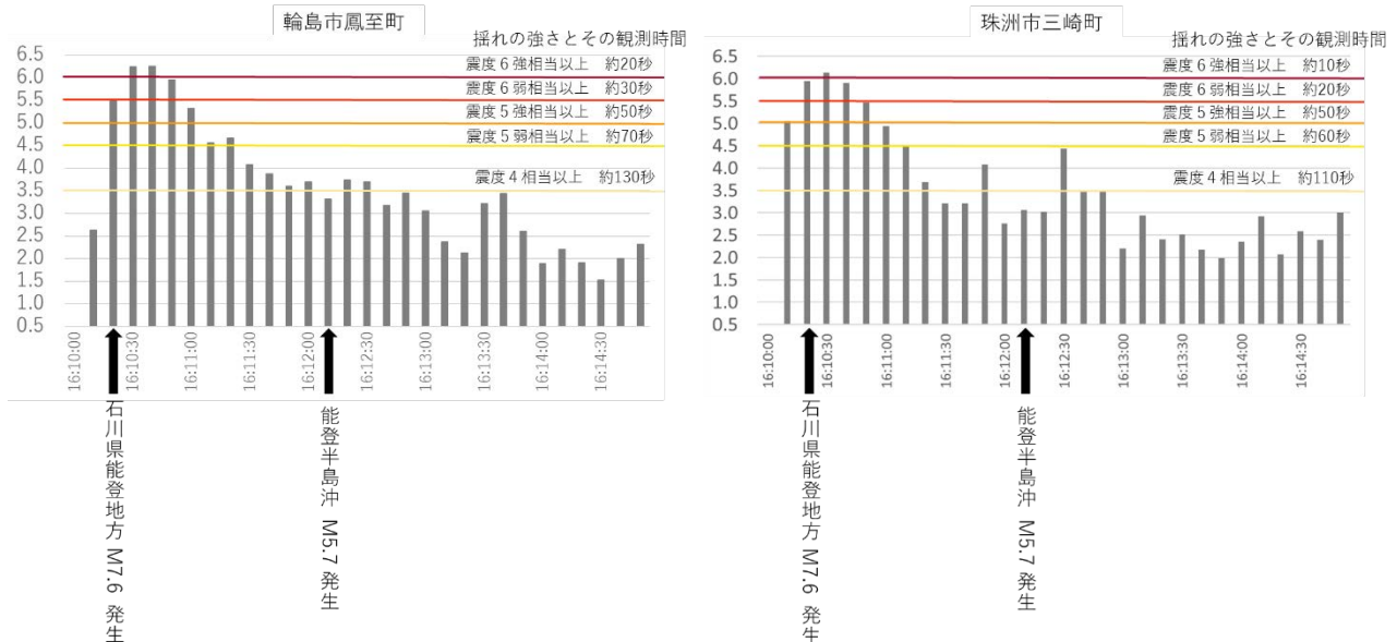
図4-1 輪島市鳳至町及び珠洲市三崎町の揺れの状況（横軸：時刻（16時10分00秒～16時15分00秒）、縦軸：通常60秒間の加速度波形から計算するものを10秒間で計算した計測震度）
