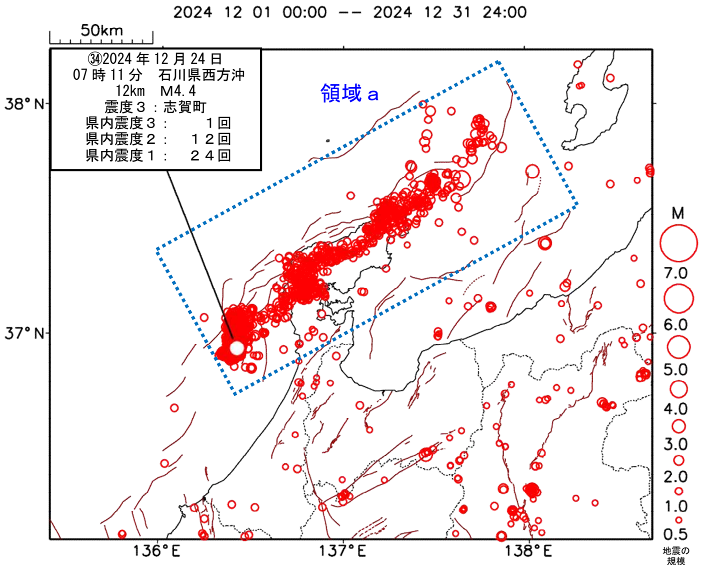
図1 令和6年（2024年）12月の深さ30km以浅、M0.5以上の地震の震央分布図 地殻内で発生した地震のみ表示している。
