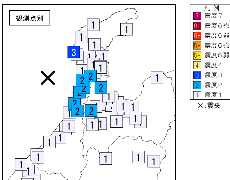
③④ 12月24日07時11分 石川県西方沖 深さ 12km M 4.4（石川県周辺）
