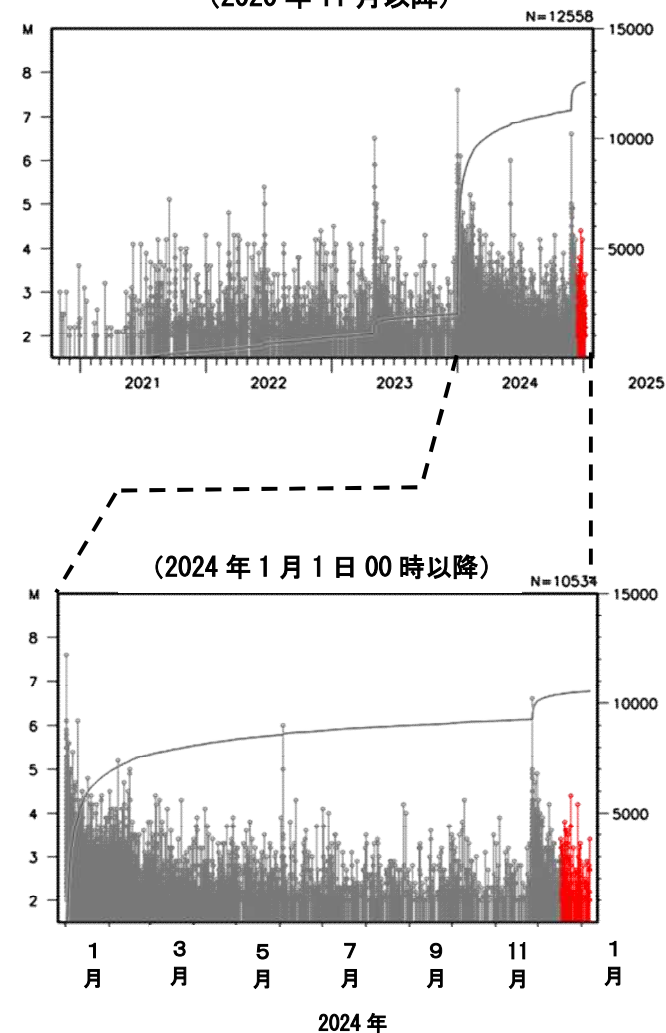
矩形領域内の地震活動経過図 (2020年11月以降)
