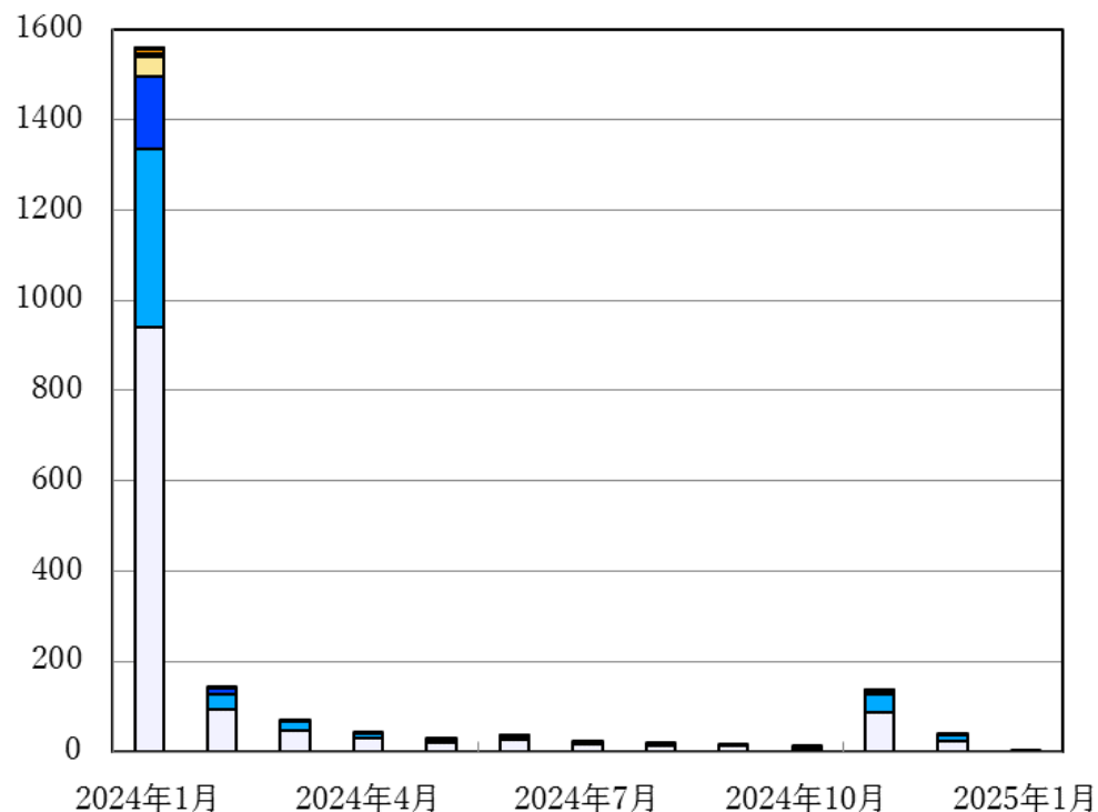
令和6年能登半島地震の地震活動による日別・震度別震度回数グラフ (2024年1月1日～2025年1月6日24時まで)
