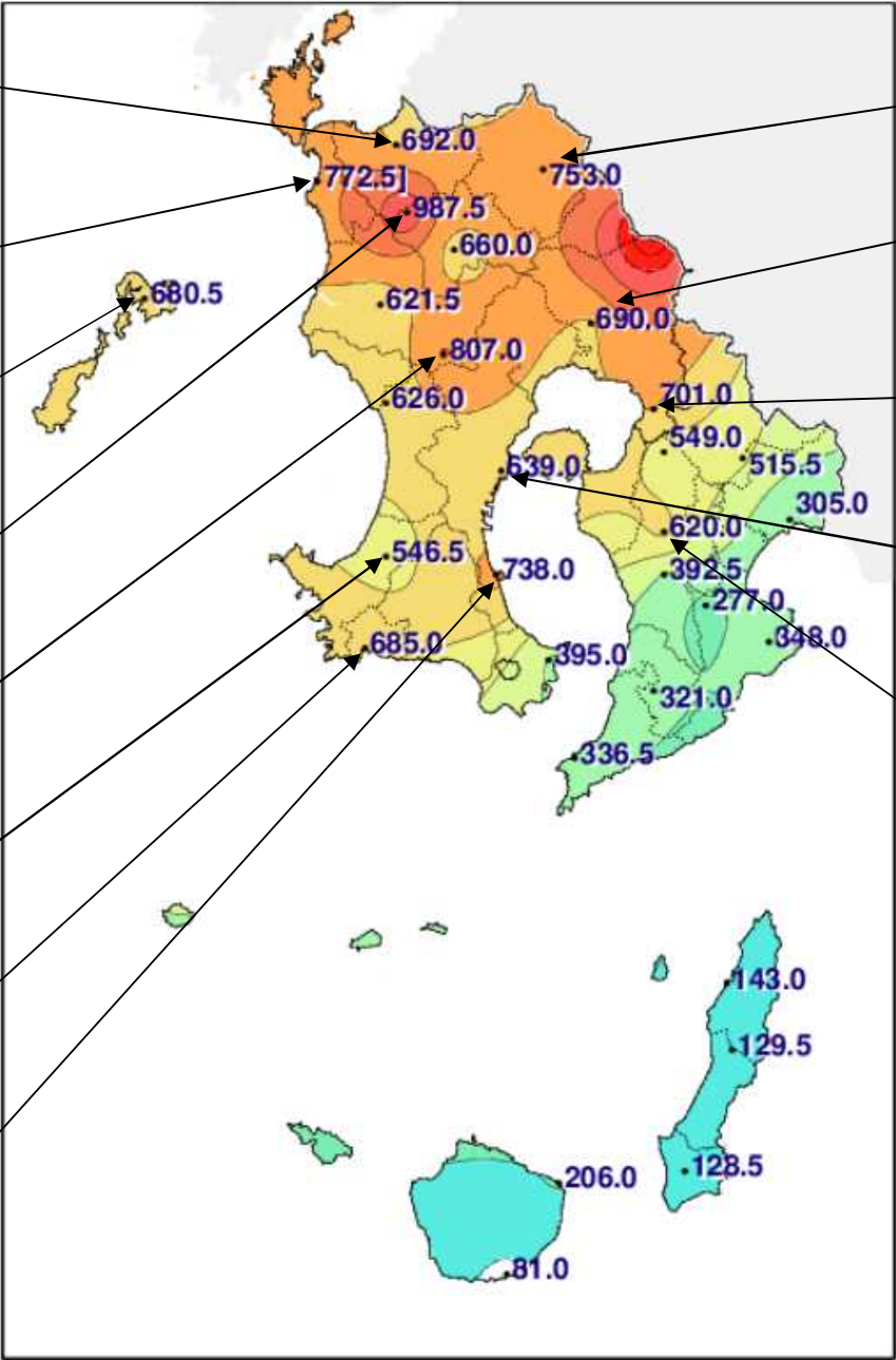
アメダス総降水量の分布図( 8月11日～19日09時)
