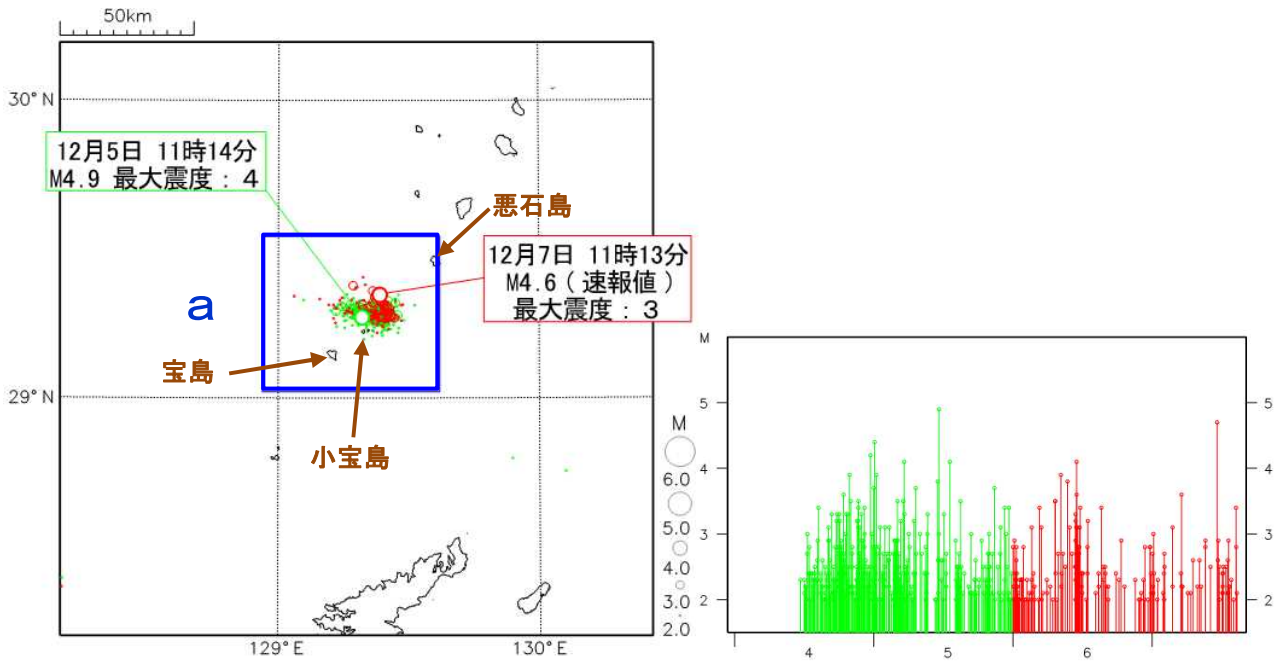
震央分布図
