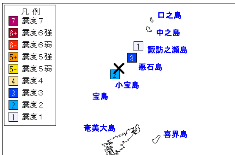
震度分布図（観測点別、×：震央） 12月7日11時13分頃 M4.6（速報値）
