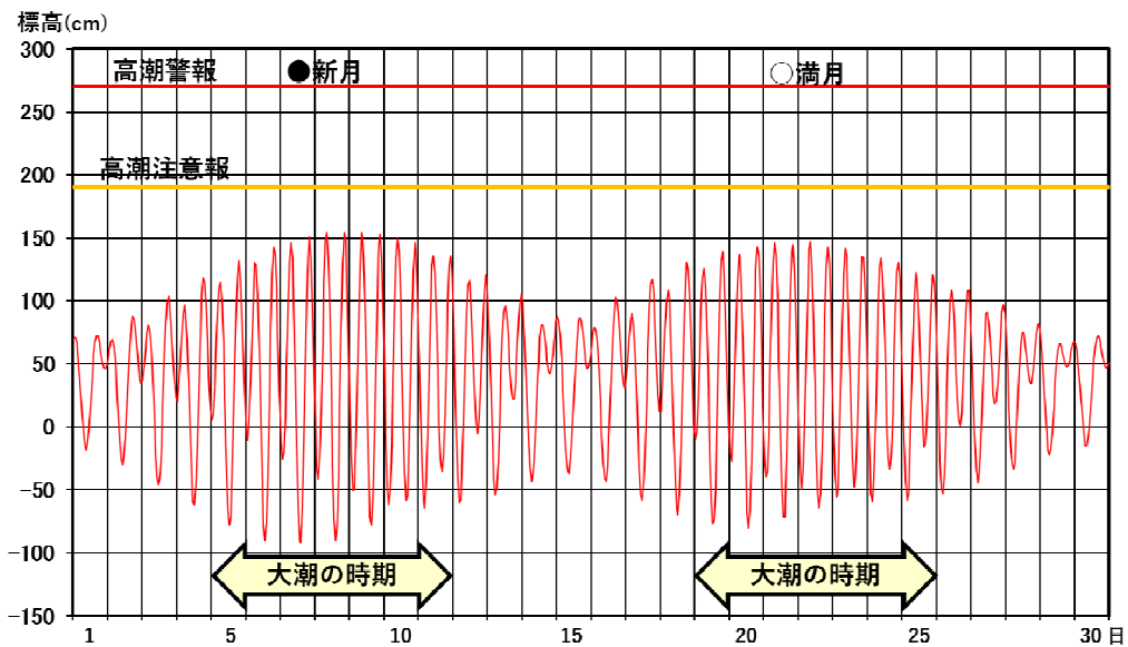
図3 枕崎における2021年9月（1時間ごとの）の天文潮位
