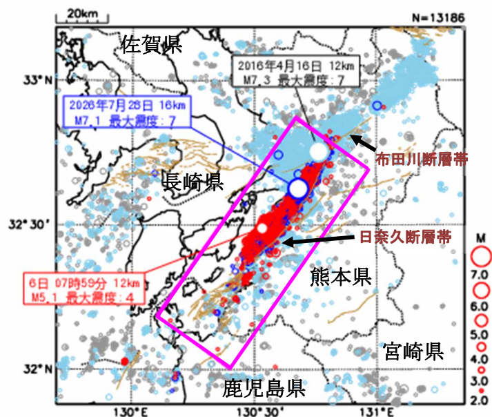
震央分布図
