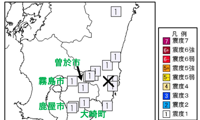
震度分布図 (観測点別、×: 震央) 23日02時07分 M3.5
