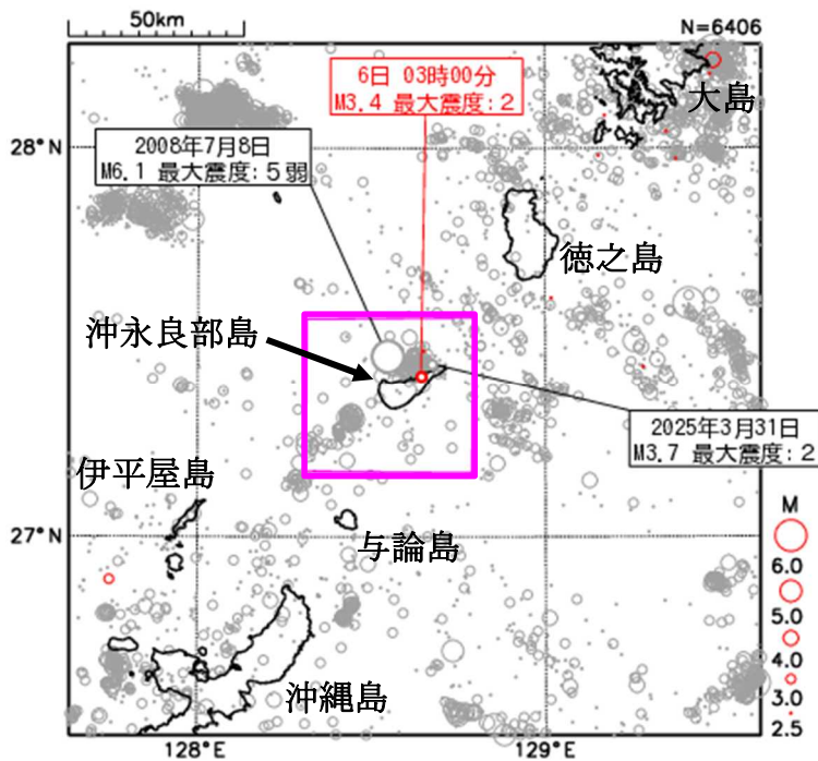
震央分布図 (1997年10月1日～2025年6月30日、 深さ0～60km、M2.5以上) 赤色は6月に発生した地震
