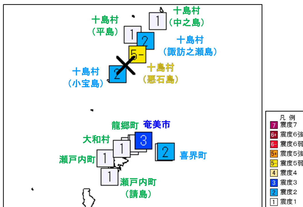
震度分布図（観測点別、×：震央） 30日18時33分 M5.3
