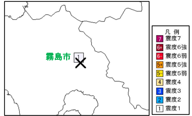
震度分布図 (観測点別、×: 震央) 22日 05時 37分 M1.5
