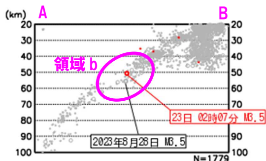
震央分布図領域aの断面図
