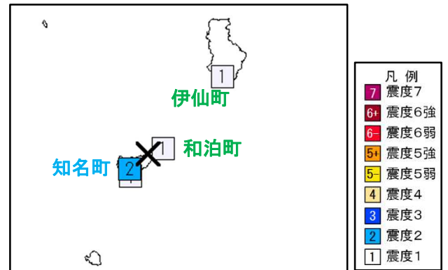
震度分布図（観測点別、×：震央） 6日03時00分 M3.4
