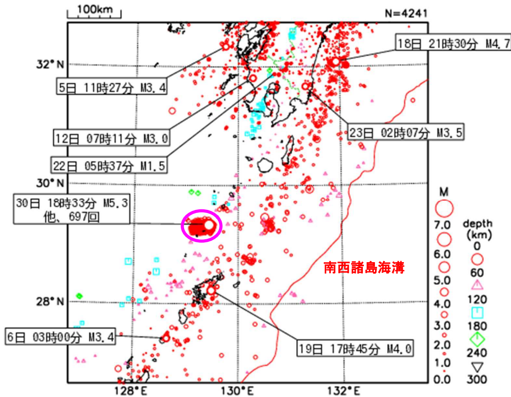
震央分布図（2025年6月1日～30日、深さ0～300km、M0.0以上）
