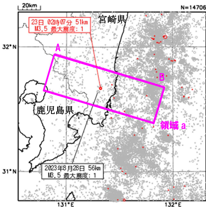
震央分布図 (1997年10月1日～2025年6月30日、 深さ20～100km、M1.5以上) 赤色は6月に発生した地震
