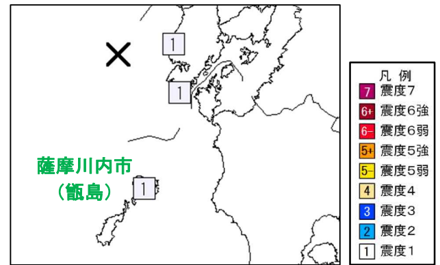
震度分布図（観測点別、×：震央） 5日 11時 27分 M3.4
