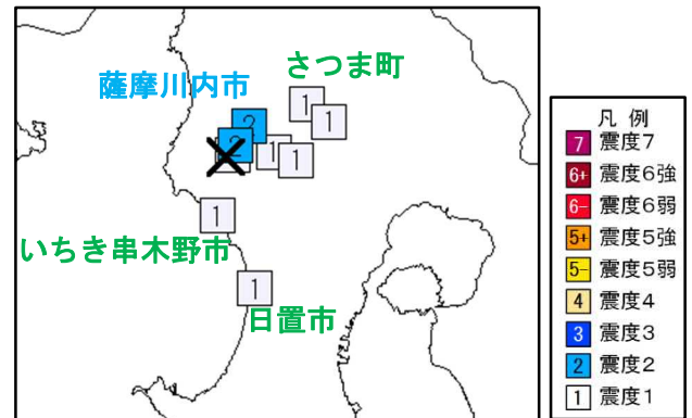
震度分布図（観測点別、×：震央） 12日07時11分 M3.0
