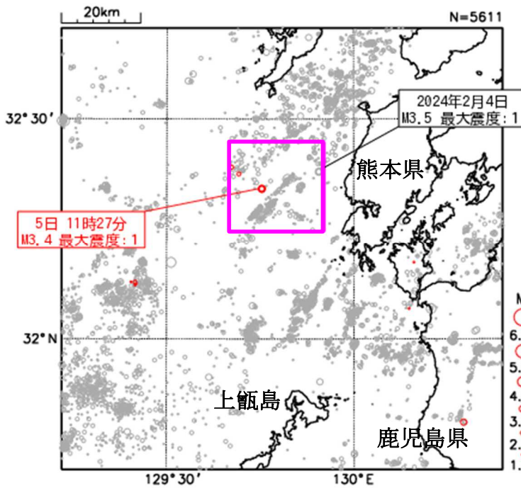
震央分布図 (2000年10月1日～2025年6月30日、 深さ0～40km、M1.5以上) 赤色は6月に発生した地震
