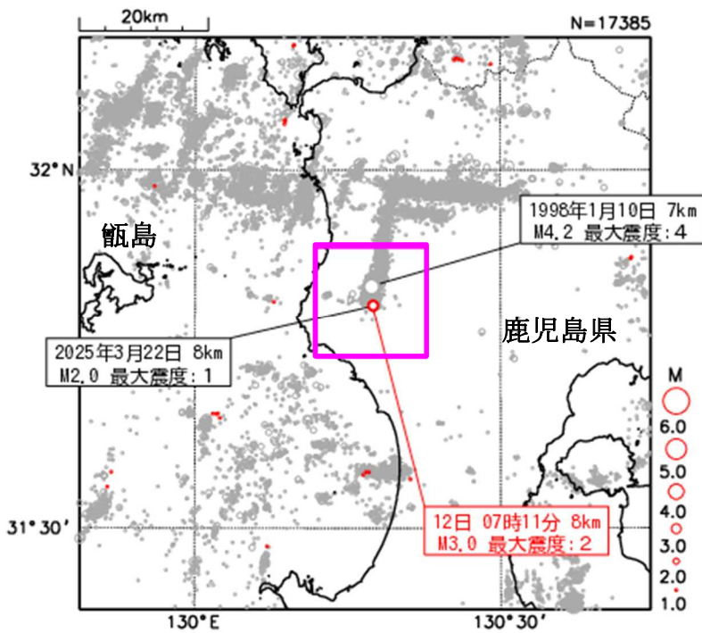
震央分布図 (1997年10月1日～2025年6月30日、 深さ0～20km、M1.0以上) 赤色は6月に発生した地震
