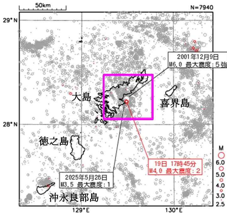
震央分布図 (1997年10月1日～2025年6月30日、 深さ0～80km、M2.5以上) 赤色は6月に発生した地震
