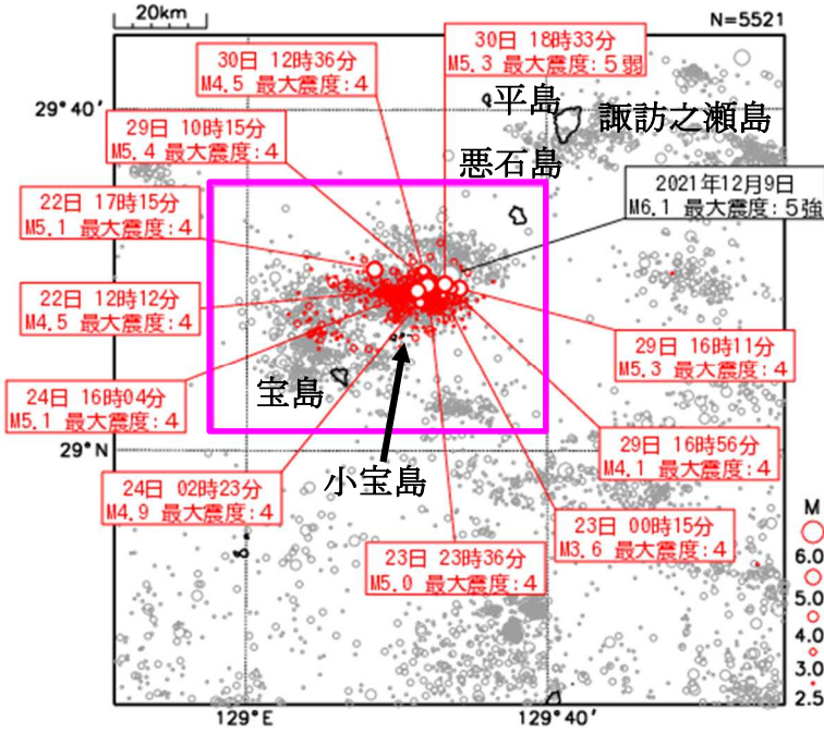
震央分布図 (1997年10月1日～2025年6月30日、 深さ0～60km、M2.5以上) 赤色は6月に発生した地震 震度4以上を観測した地震に吹出しを付加
