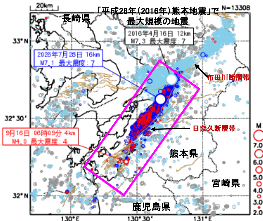
震央分布図
