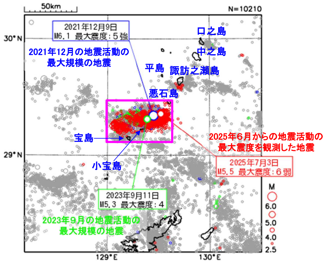
震央分布図
