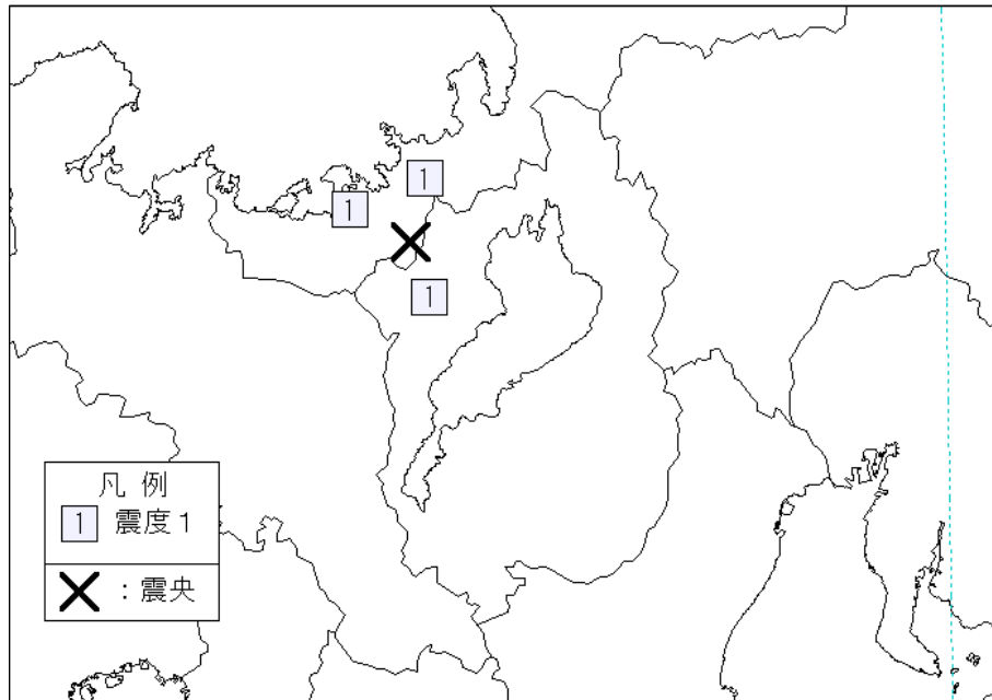
各観測点の震度
