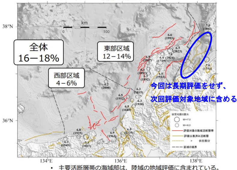
評価対象海域の各区域における今後30年以内に M7.0以上の地震が発生する確率
