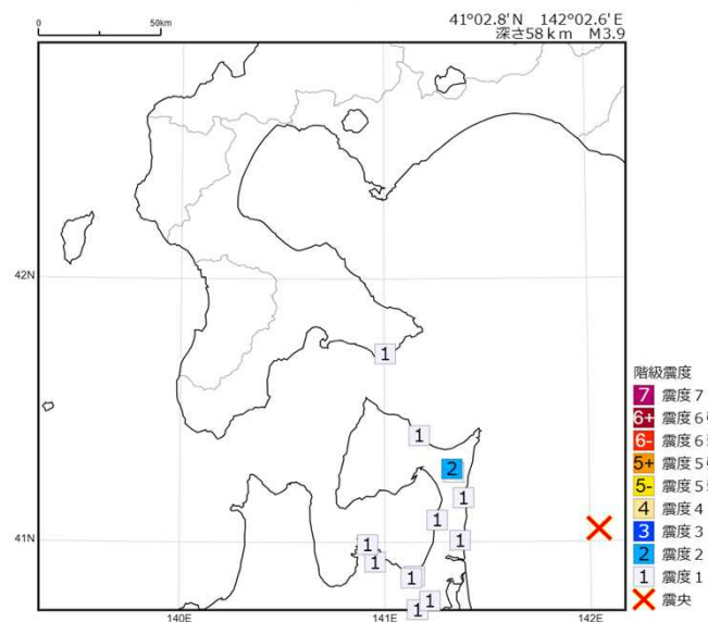
2025年 9月 6日 12時48分 青森県東方沖の地震の震度分布図
