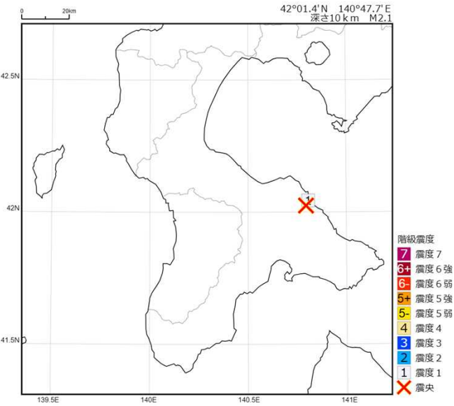
2025年 9月25日 01時50分 渡島地方東部の地震の震度分布図
