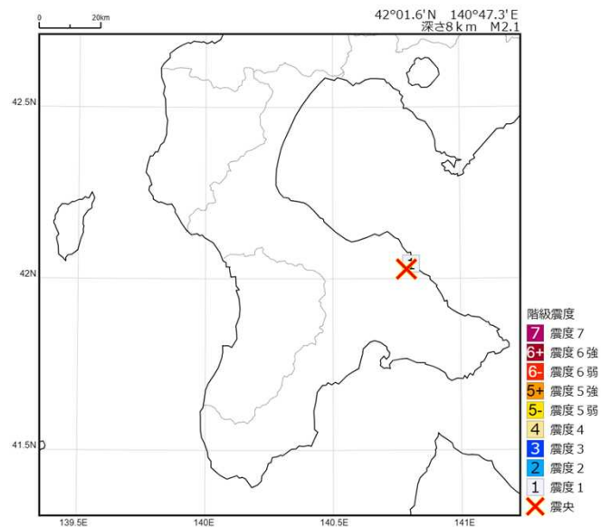
2025年 9月23日 19時05分 渡島地方東部の地震の震度分布図
