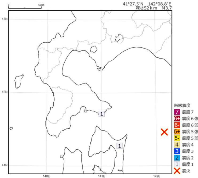
2025年 9月28日 11時45分 青森県東方沖の地震の震度分布図
