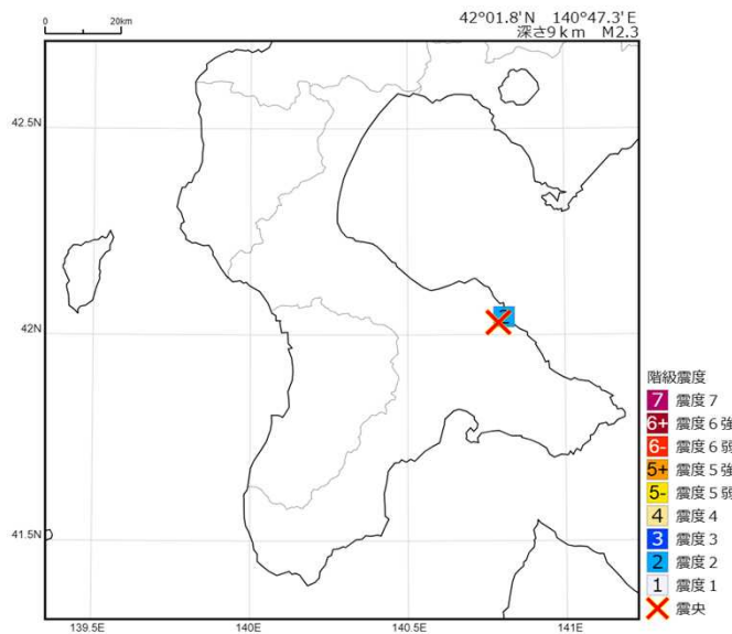
2025年 9月23日 16時37分 渡島地方東部の地震の震度分布図
