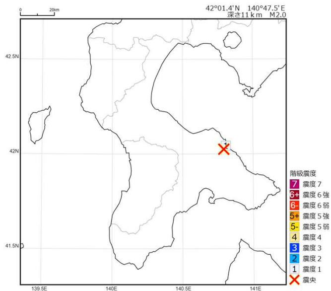
2025年 9月23日 18時57分 渡島地方東部の地震の震度分布図
