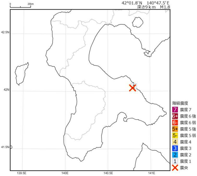
2025年 9月25日 13時20分 渡島地方東部の地震の震度分布図
