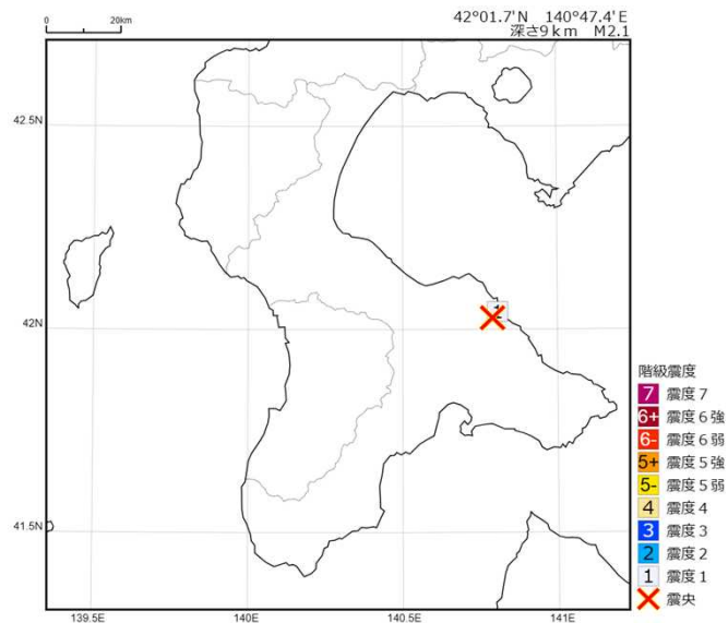
2025年 9月23日 22時43分 渡島地方東部の地震の震度分布図
