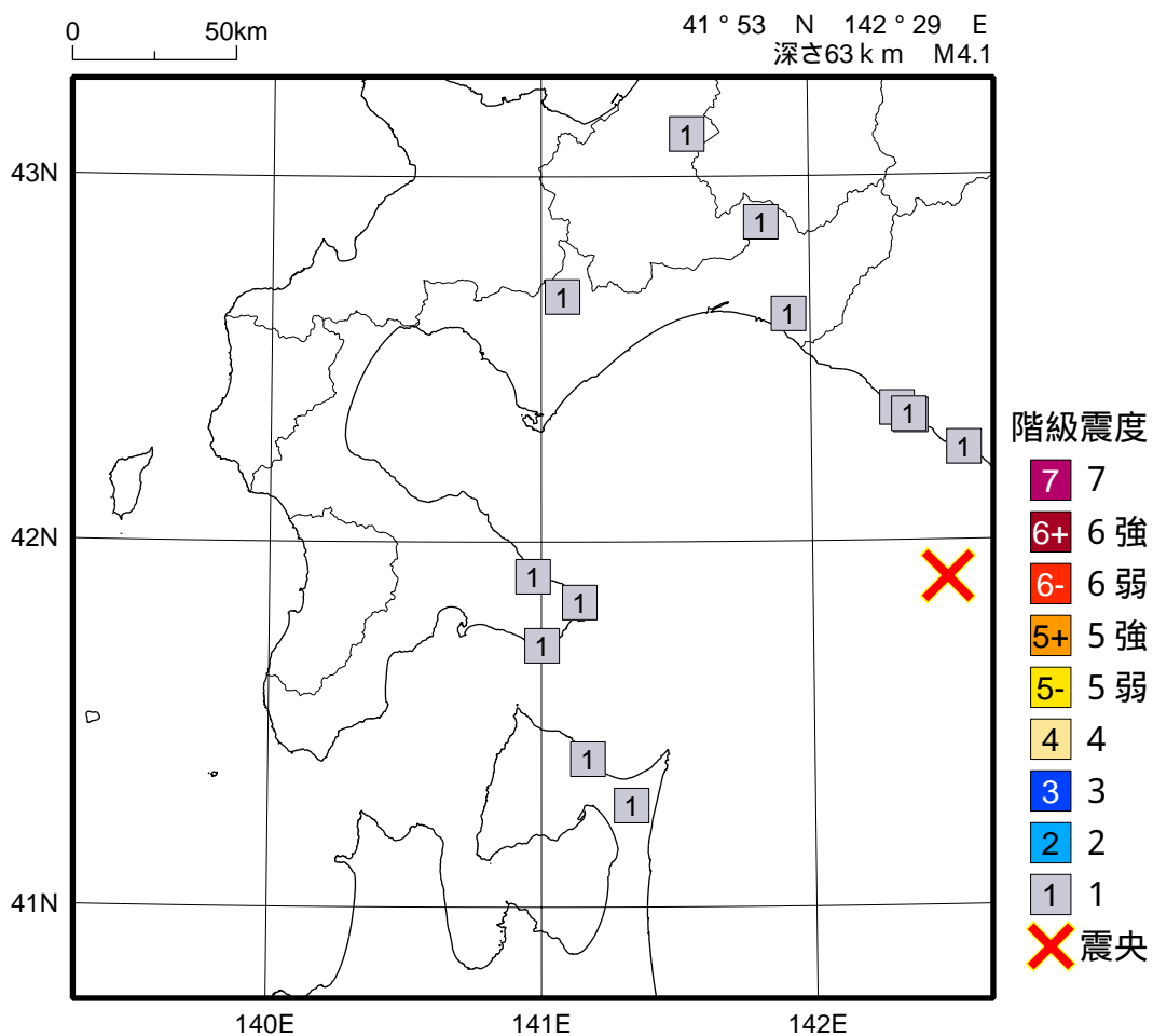
2021年 7月 4日02時19分 浦河沖の地震の震度分布図
