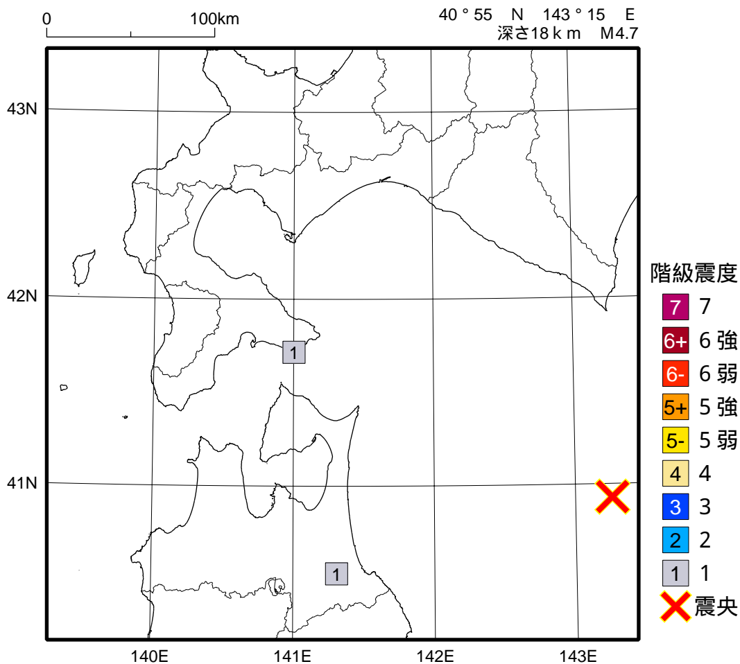
2020年11月 6日18時17分 青森県東方沖の地震の震度分布図
