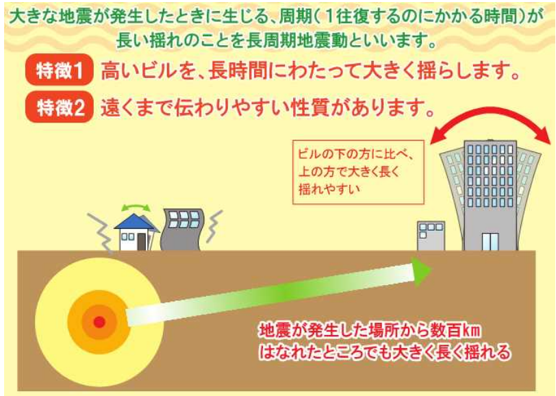
図1 長周期地震動の概要と特徴
