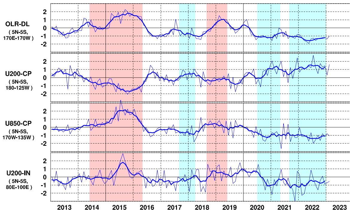
図 8 日付変更線付近の OLR 指数 (OLR-DL)、対流圏上層 (200hPa) の赤道東西風指数 (U200-CP)、対 流圏下層 (850hPa) の赤道東西風指数 (U850-CP)、インド洋における対流圏上層 (200hPa) の赤道東西風指数 (U200-IN) の時系列 (上から順に) 折線は月平均値、滑らかな太線は 5 か月移動平均値を示す (平年値は 1991~2020 年の 30 年平均値)。赤色の陰影はエル ニニョ現象の発生期間を、青色の陰影はラニーニャ現象の発生期間を示している。
