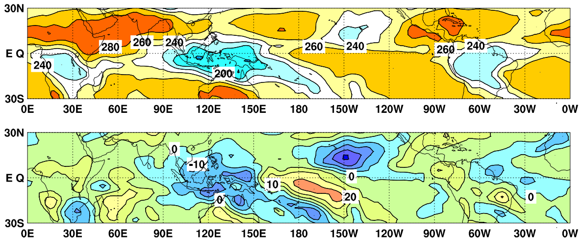
図9 外向き長波放射量 (OLR) (上) 及び平年偏差 (下) の分布図 (2023年2月)
