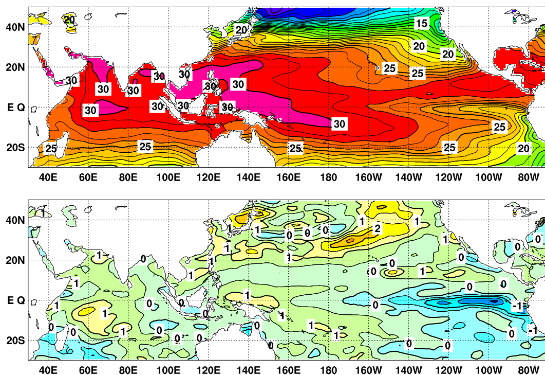
図4 2020年6月の海面水温図(上)及び平年偏差図(下)
