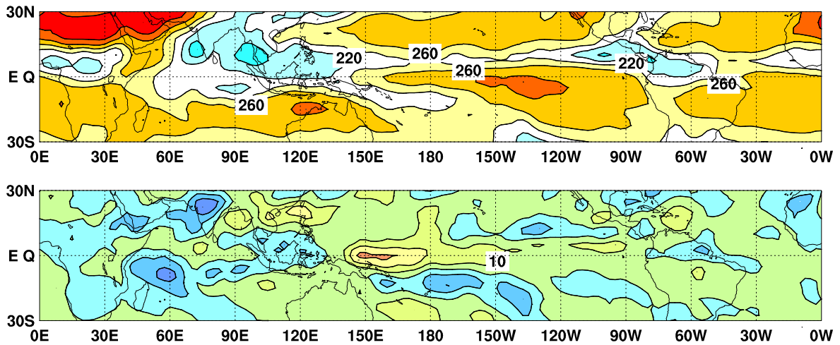
図9 外向き長波放射量 (OLR) (上) 及び平年偏差 (下) の分布図 (2020年6月)
