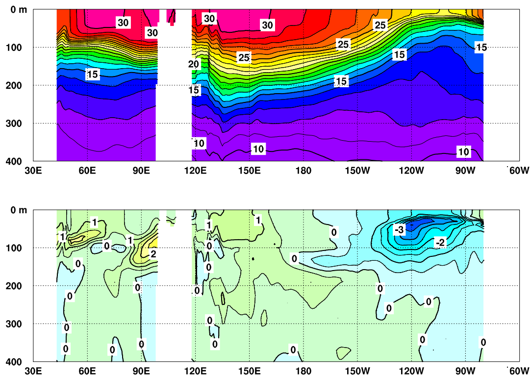
図5 2020年6月のインド洋から太平洋の赤道に沿った水温(上)及び平年偏差(下)の断面図
