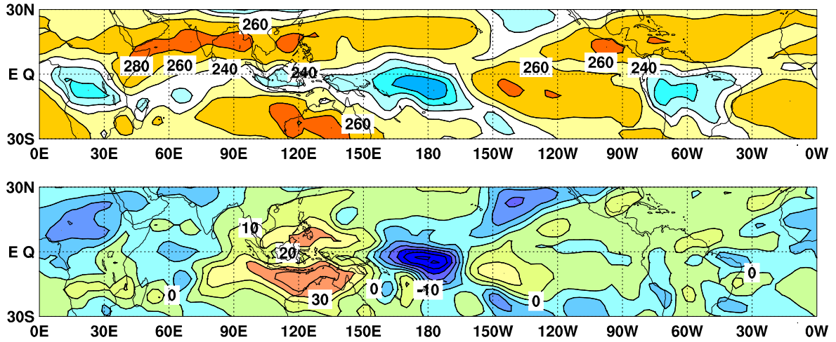
図9 外向き長波放射量 (OLR) (上) 及び平年偏差 (下) の分布図 (2019年2月)
