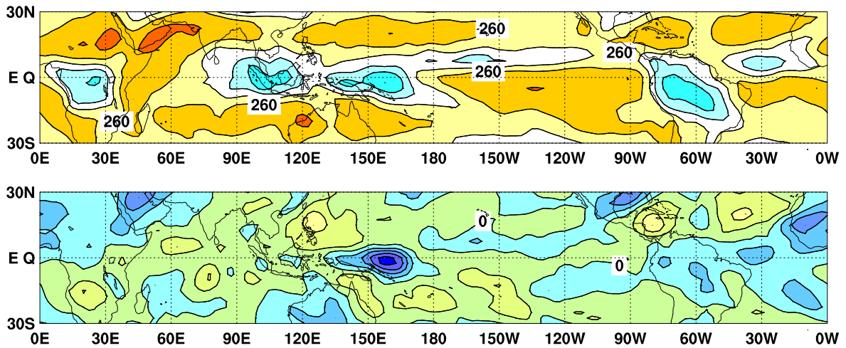
図9 外向き長波放射量 (OLR) (上) 及び年偏差 (下) の分布図 (2018年11月)
