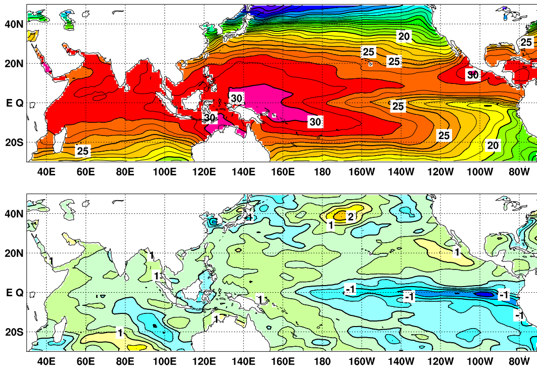
図4 2017年11月の海面水温図（上）及び平年偏差図（下）
