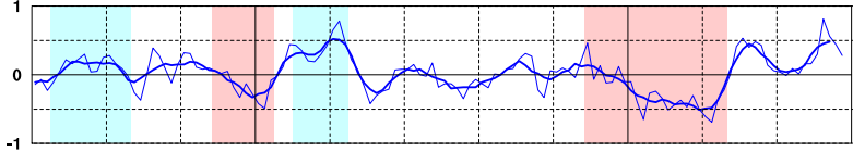
(c) 西太平洋熱帯域の海面水温の基準値*との差 ( ^{\circ}\text{C} )
