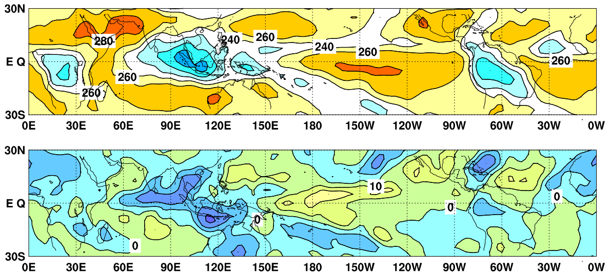
図 8 外向き長波放射量 (OLR) (上) 及び年偏差 (下) の分布図 (2017 年 11 月)
