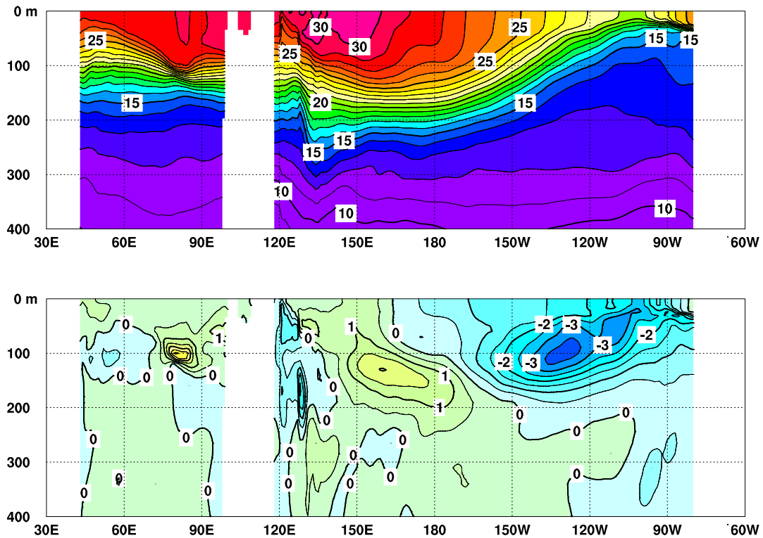
図5 2017年11月のインド洋から太平洋の赤道に沿った水温（上）及び平年偏差（下）の断面図
