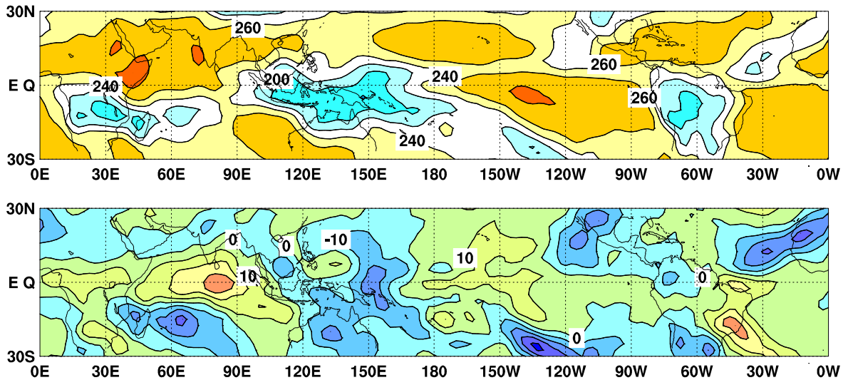
図6 外向き長波放射量 (OLR) (上) 及び年偏差 (下) の分布図 (2015 年 1 月)
