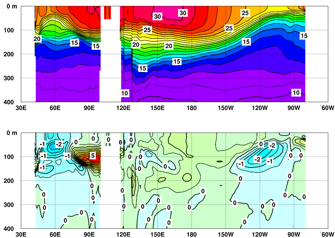
図 3 2015 年 1 月のインド洋から太平洋の赤道に沿った水温 ( 上 ) 及び平年偏差 ( 下 ) の断面図
