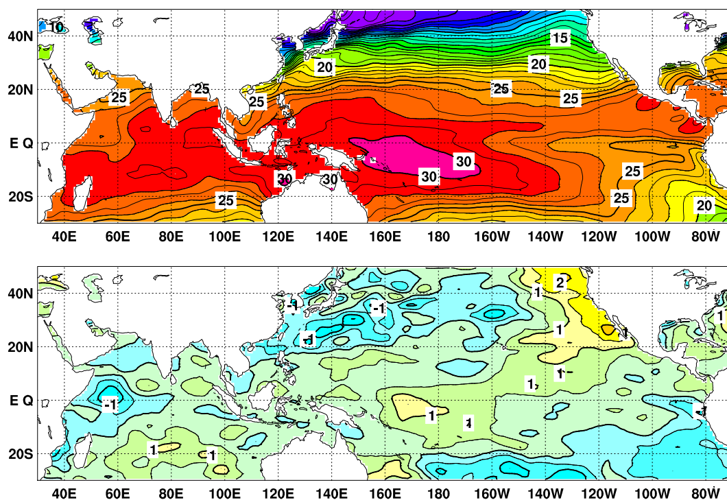
図 2 2015 年 1 月の海面水温図 ( 上 ) 及び平年偏差図 ( 下 )
