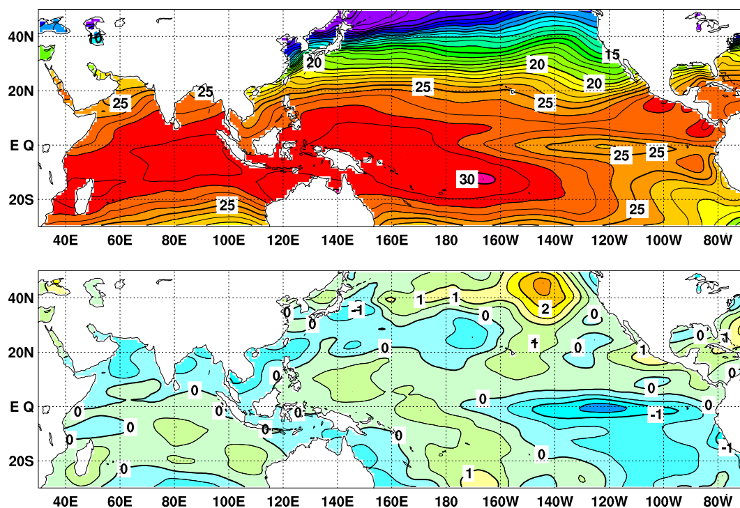
図 2 2014 年 2 月の海面水温図 ( 上 ) 及び平年偏差図 ( 下 )
