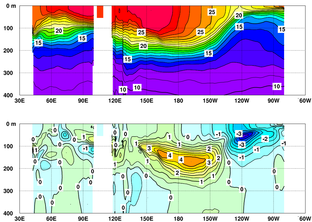
図 3 2014 年 2 月のインド洋から太平洋の赤道に沿った水温 ( 上 ) 及び平年偏差 ( 下 ) の断面図
