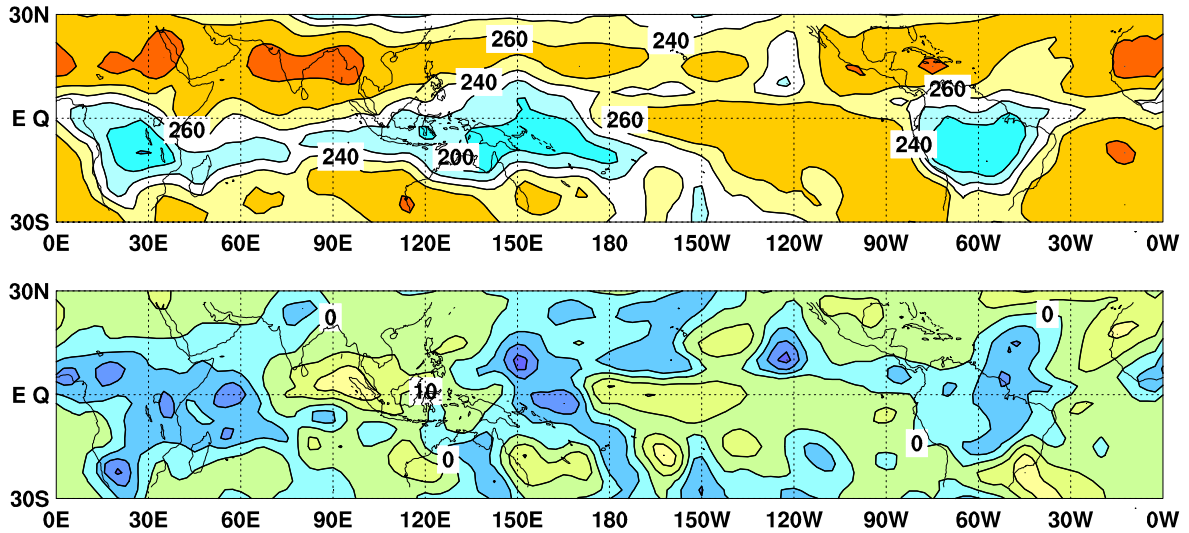
図 6 外向き長波放射量 (OLR) (上) 及び年偏差 (下) の分布図 (2014 年 2 月)
