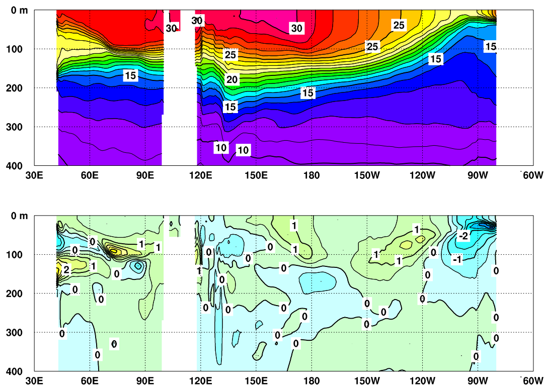
図 3 2012 年 11 月のインド洋から太平洋の赤道に沿った水温 ( 上 ) 及び平年偏差 ( 下 ) の断面図
