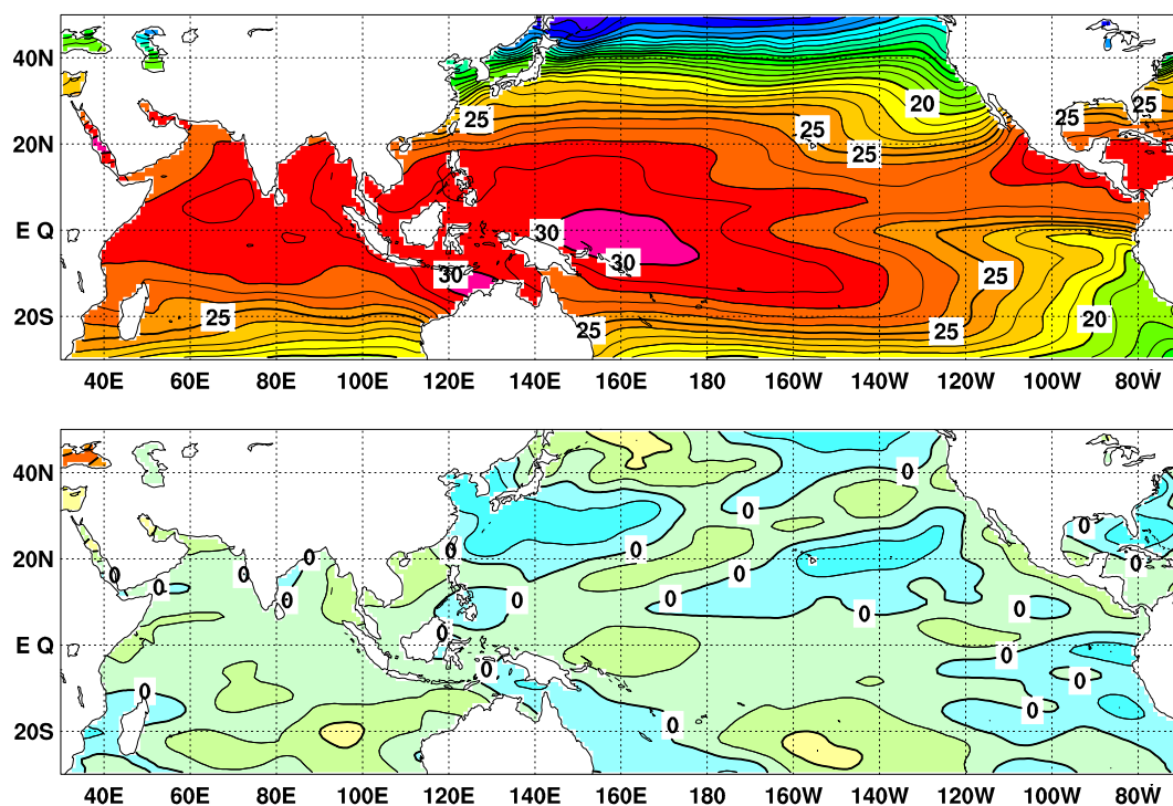
図 2 2012 年 11 月の海面水温図 ( 上 ) 及び平年偏差図 ( 下 )
