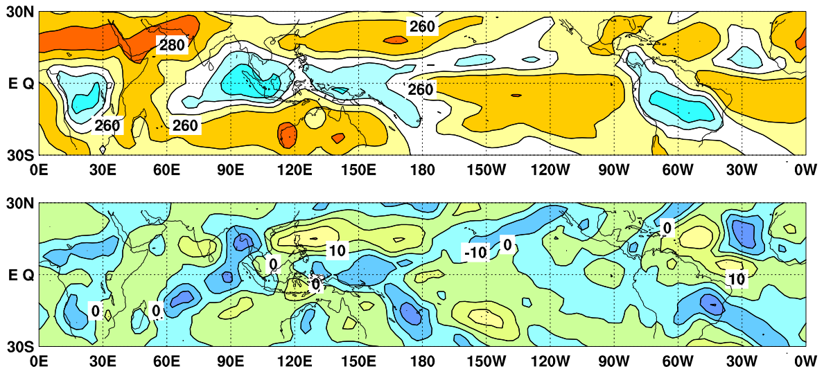
図6 外向き長波放射量 (OLR) (上) 及び年偏差 (下) の分布図 (2012年11月)
