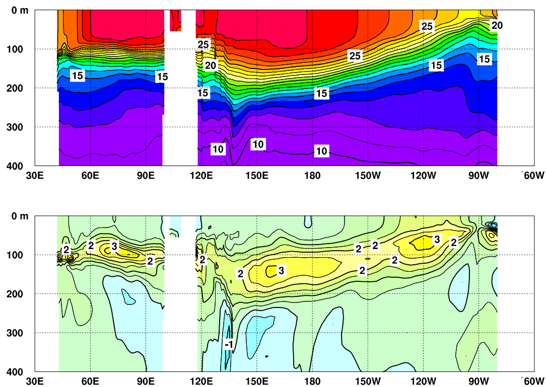
図 3 2012 年 7 月のインド洋から太平洋の赤道に沿った水温 ( 上 ) 及び平年偏差 ( 下 ) の断面図
