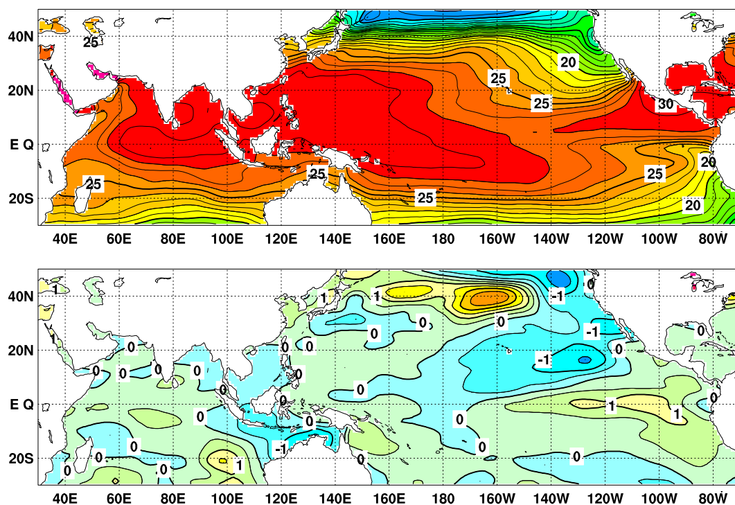
図 2 2012 年 7 月の海面水温図 ( 上 ) 及び平年偏差図 ( 下 )
