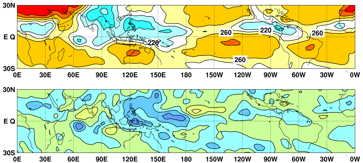
図6 外向き長波放射量(OLR)(上)及び年偏差(下)の分布図(2012年7月)
