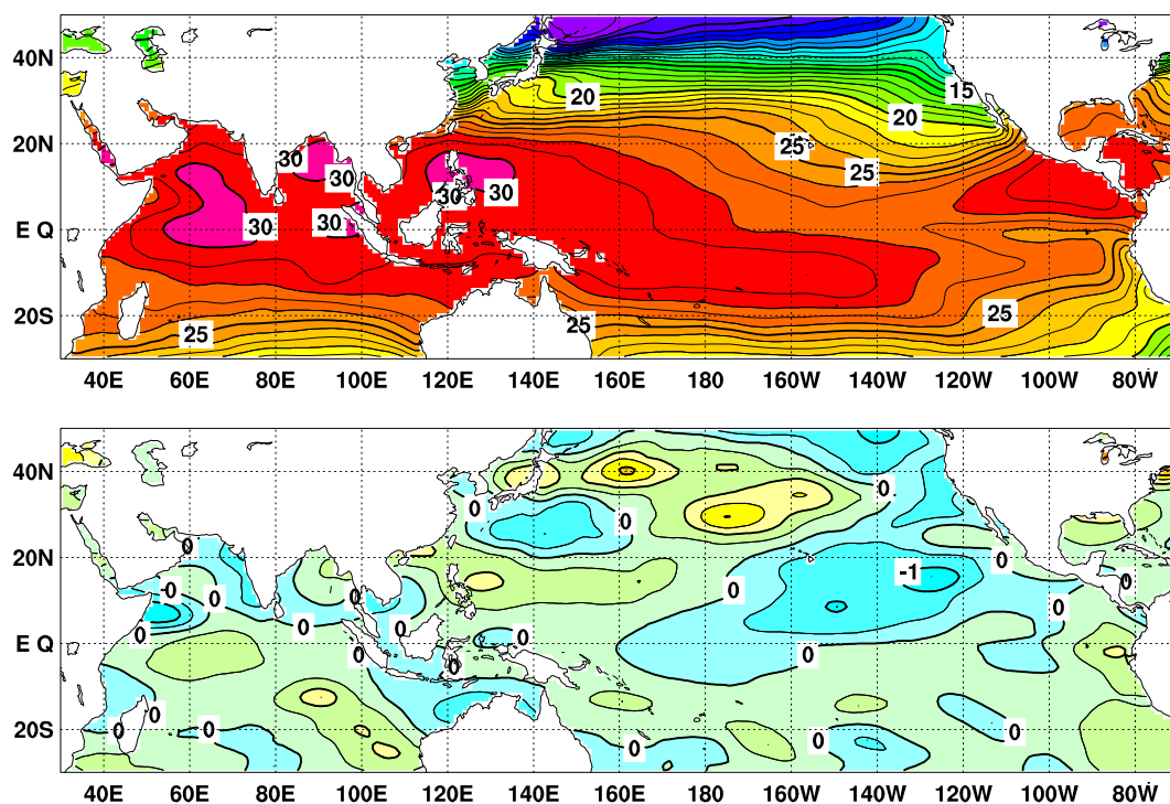
図 2 2012 年 5 月の海面水温図 ( 上 ) 及び平年偏差図 ( 下 )
