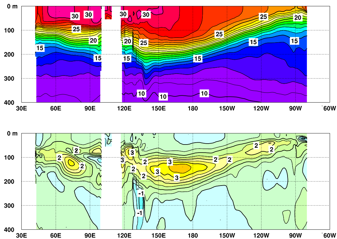
図 3 2012 年 5 月のインド洋から太平洋の赤道に沿った水温 ( 上 ) 及び平年偏差 ( 下 ) の断面図
