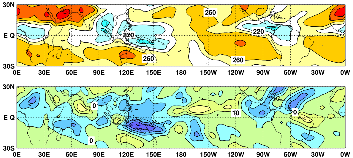
図6 外向き長波放射量 ( OLR ) ( 上 ) 及び平年偏差 ( 下 ) の分布図 ( 2012 年 5 月 )
