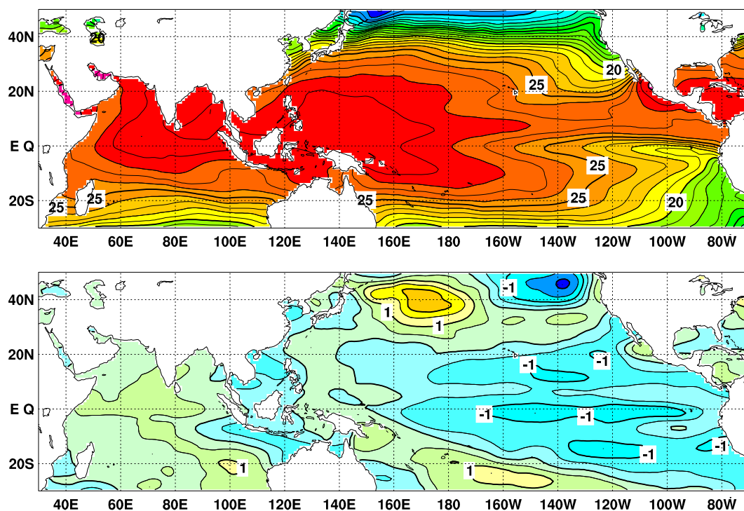
図 2 2011 年 10 月の海面水温図 ( 上 ) 及び平年偏差図 ( 下 )
