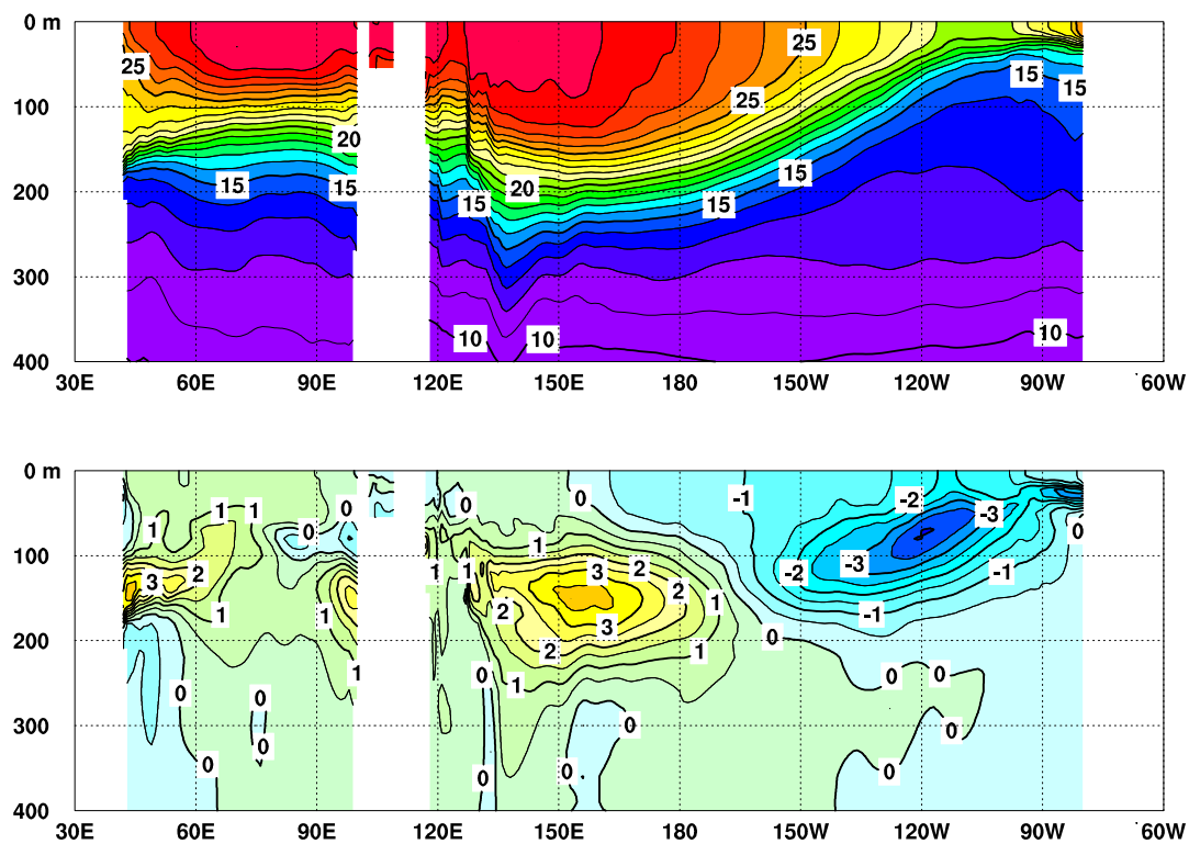
図 3 2011 年 10 月のインド洋から太平洋の赤道に沿った水温 ( 上 ) 及び平年偏差 ( 下 ) の断面図
