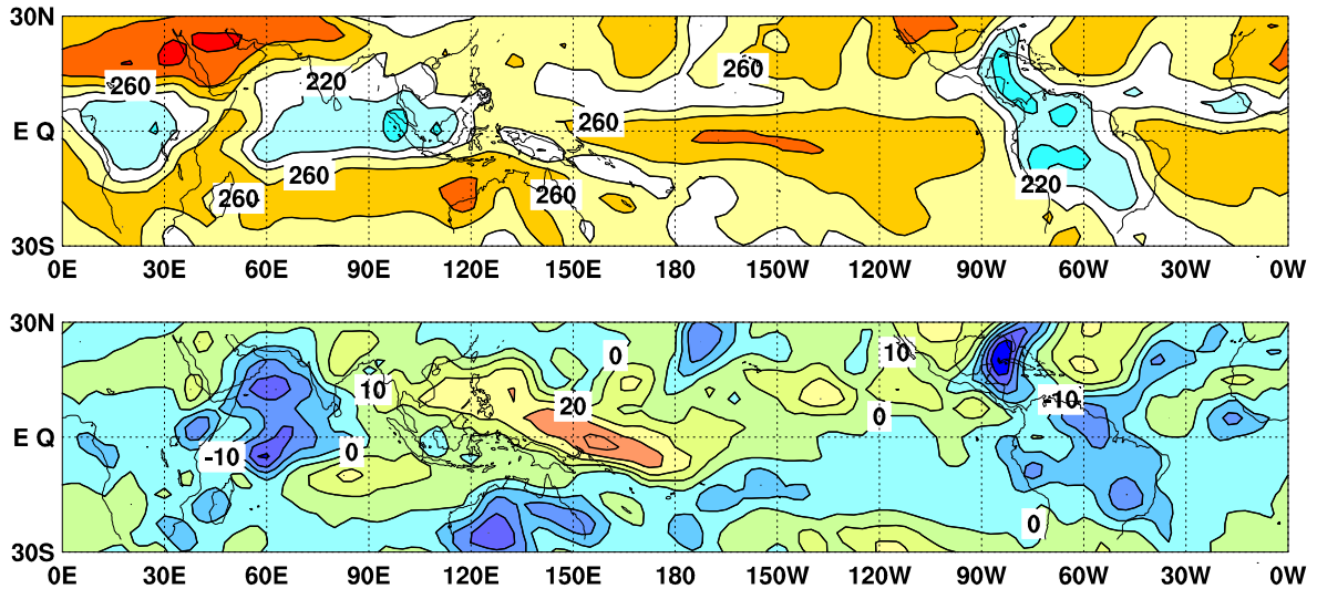
図6 外向き長波放射量 (OLR) (上) 及び年偏差 (下) の分布図 (2011 年 10 月)
