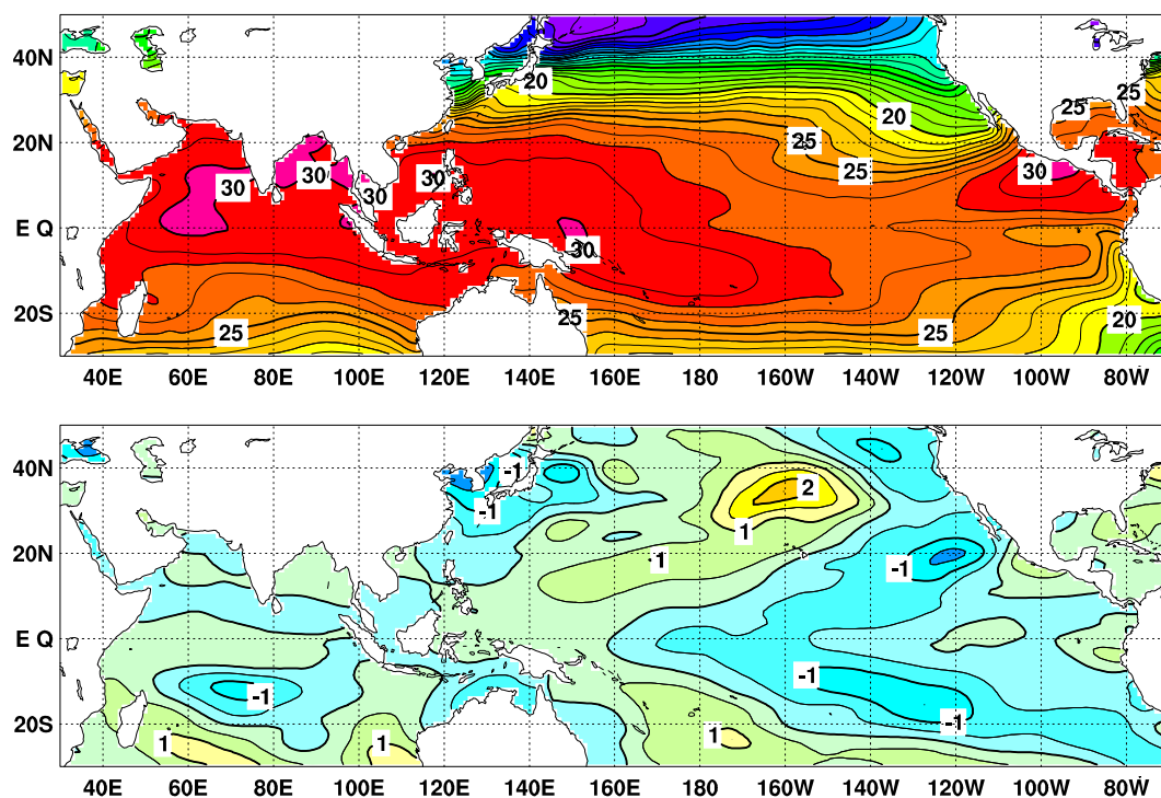
図 2 2011 年 5 月の海面水温図 ( 上 ) 及び 平年偏差図 ( 下 )
