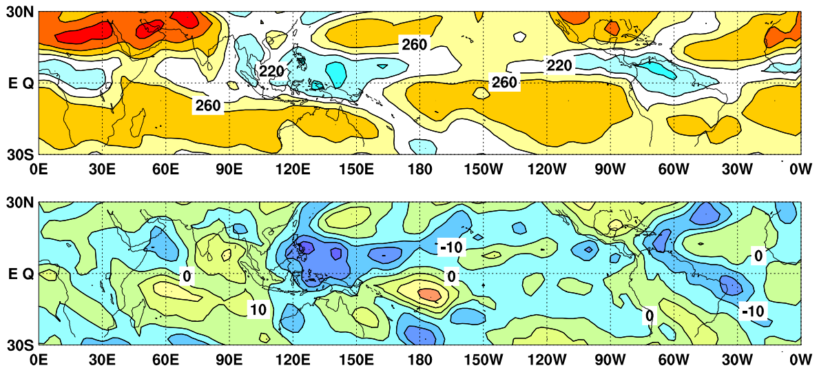
図 6 外向き長波放射量 (OLR) (上) 及び年偏差 (下) の分布図 (2011 年 5 月)
