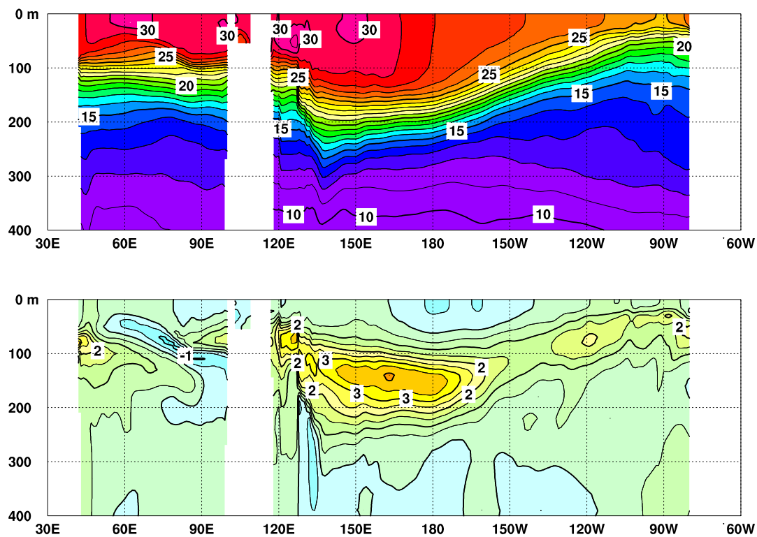
図 3 2011 年 5 月のインド洋から太平洋の赤道に沿った水温 ( 上 ) 及び 平年偏差 ( 下 ) の断面図
