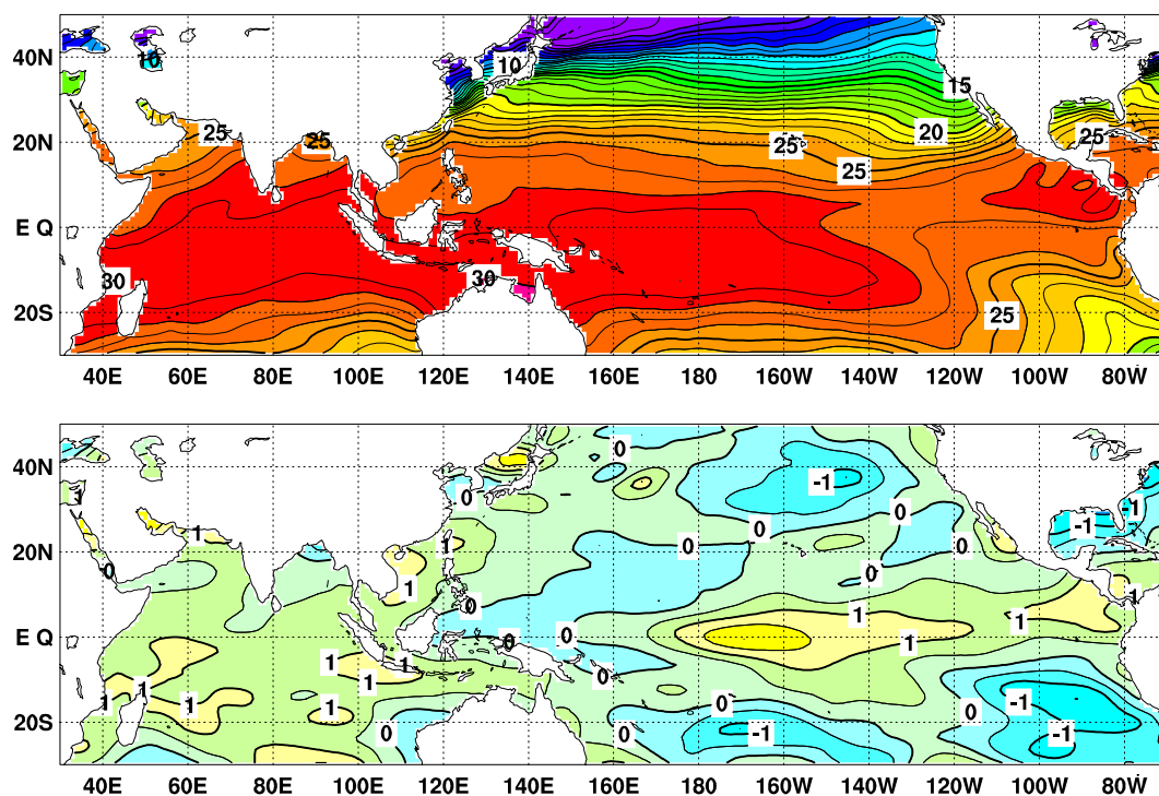
図 2 2010 年 2 月の海面水温図 ( 上 ) 及び 年 平 均 偏 差 図 ( 下 )
