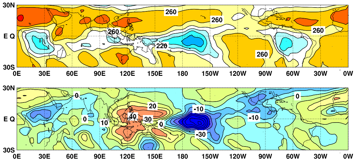
図6 外向き長波放射量 (OLR) (上) 及び年偏差 (下) の分布図 (2010 年 2 月)
