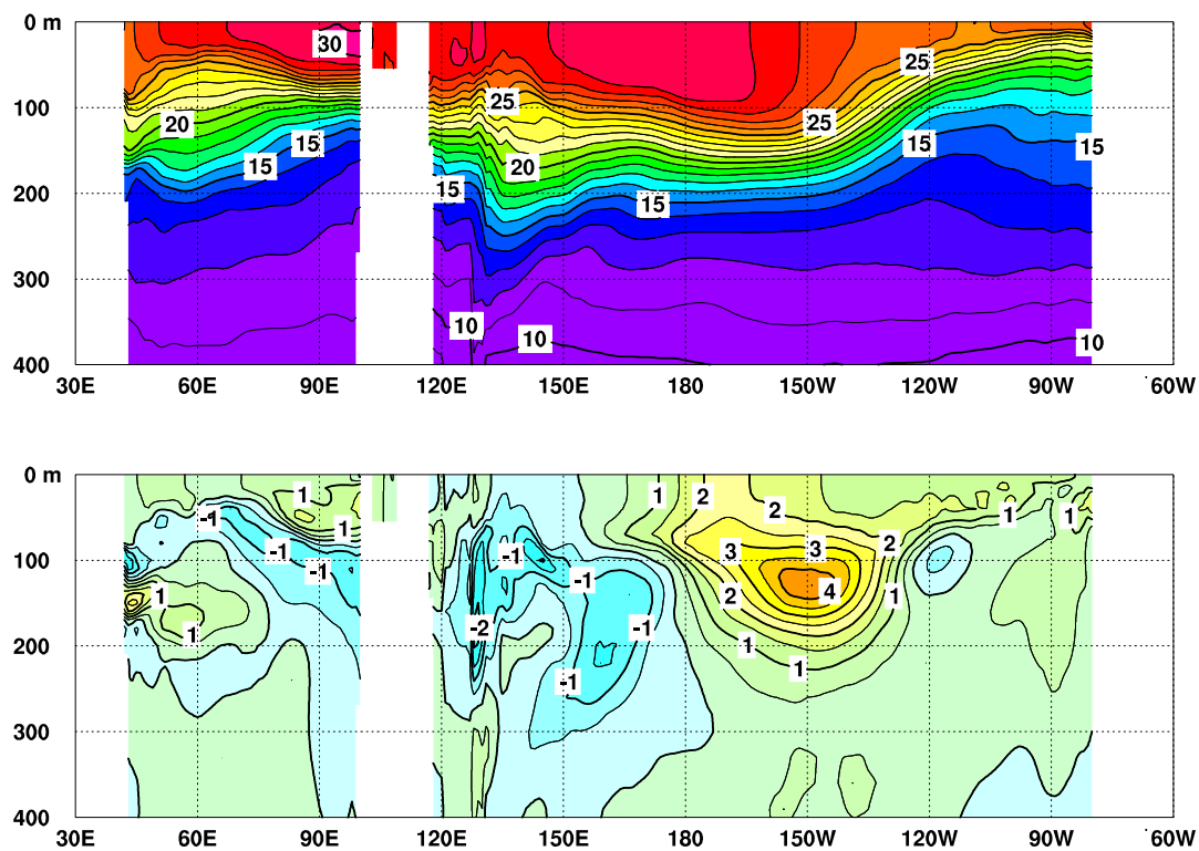
図 3 2010 年 2 月の イ ン ド 洋 か ら 太 平 洋 の 赤 道 に 沿 っ た 水 温 ( 上 ) 及 び 年 平 均 偏 差 ( 下 ) の 断 面 図
