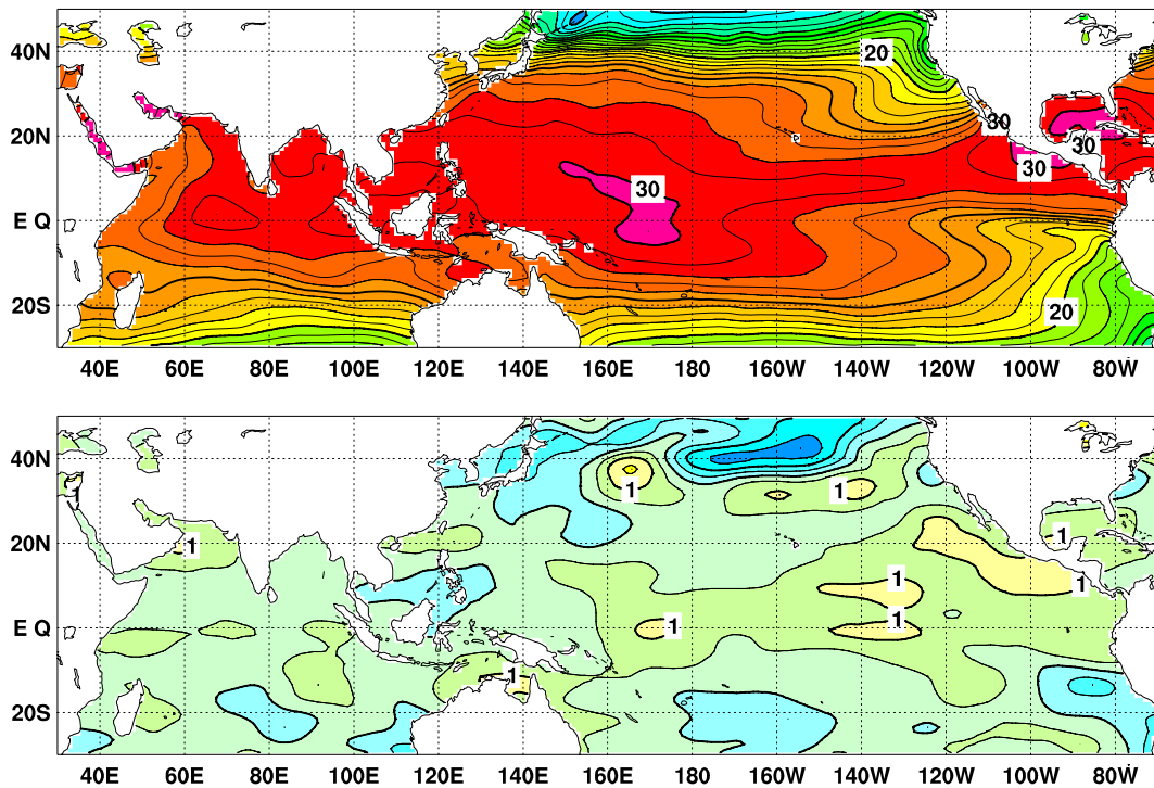
図 2 2009 年 9 月の海面水温図 ( 上 ) 及び 年 平 均 偏 差 図 ( 下 )
