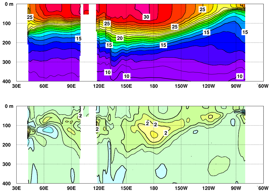
図 3 2009 年 9 月のインド洋から太平洋の赤道に沿った水温 ( 上 ) 及び 年 平 均 偏 差 ( 下 ) の 断 面 図
