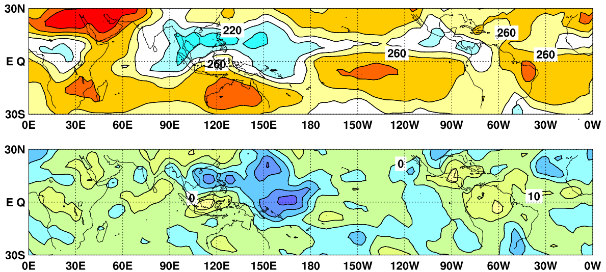
図6 外向き長波放射量 (OLR) (上) 及び年偏差 (下) の分布図 (2009 年 9 月)
