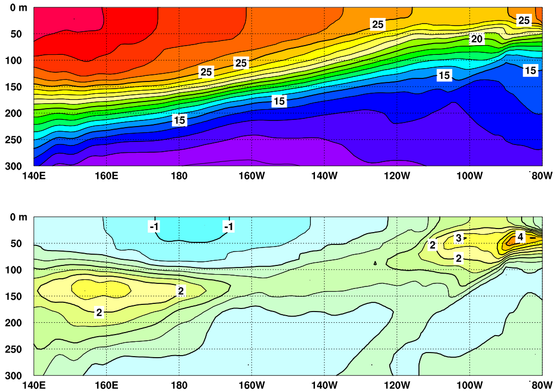
図3 2008年6月の太平洋の赤道に沿った水温(上)及び平年偏差(下)の断面図(海洋データ同化システムによる)。上図の等値線間隔は 1^{\circ}\text{C} 、下図の等値線間隔は 0.5^{\circ}\text{C} (平年値は1979~2004年の26年平均値)。
