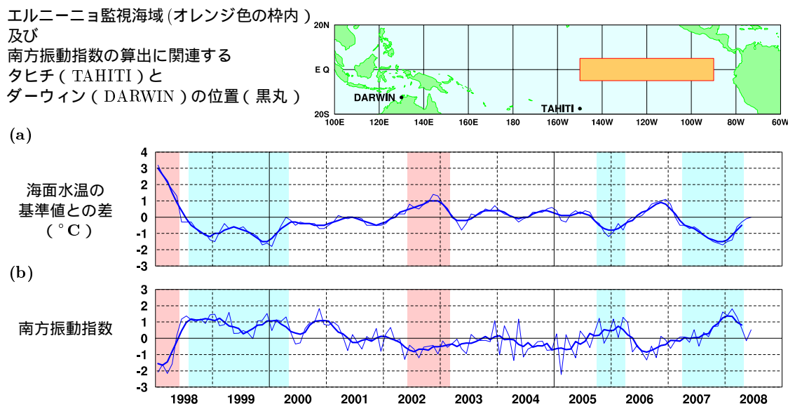
図1 エルニーニョ監視海域の海面水温の基準値との差( ^{\circ}\text{C} )(a)と南方振動指数(b)の推移(1998年1月~2008年6月)。折線は月平均値、滑らかな太線は5か月移動平均値を示す(海面水温の基準値はその年の前年までの30年間の各月の平均値、南方振動指数の年平均値は1971~2000年の30年平均値)。赤色の陰影はエルニーニョ現象の発生期間を、青色の陰影はラニーニャ現象の発生期間を示している。
