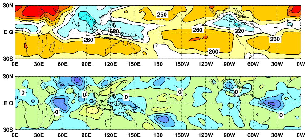
図 6 2008 年 6 月の外向き長波放射量 (OLR) ( 上 ) 及び平年偏差 ( 下 ) の分布図。OLR の値が小さいほど、対流活動が活発であることを示す。上図は 20\text{W}/\text{m}^2 毎、下図は 10\text{W}/\text{m}^2 毎に等値線を描いている ( 平年値は 1979 ~ 2004 年の 26 年平均値 )。OLR データは米国海洋大気庁 ( NOAA ) から提供されたものである。
