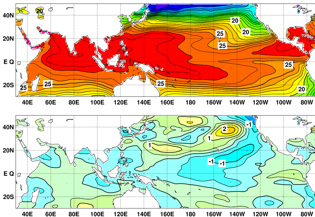
図 2 2008 年 6 月の海面水温図 ( 上 ) 及び平年偏差図 ( 下 )。海面水温図の太線は 5^{\circ}\text{C} 毎、細線は 1^{\circ}\text{C} 毎の、平年偏差図の太線は 1^{\circ}\text{C} 毎、細線は 0.5^{\circ}\text{C} 毎の等値線を示す ( 平年値は 1971 ~ 2000 年の 30 年平均値 )。
