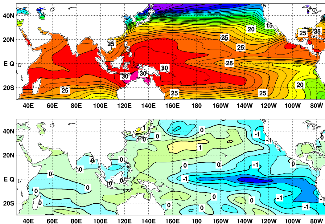
図 2 2007 年 12 月の海面水温図 ( 上 ) 及び平年偏差図 ( 下 )、海面水温図の太線は 5^{\circ}\text{C} 毎、細線は 1^{\circ}\text{C} 毎の、平年偏差図の太線は 1^{\circ}\text{C} 毎、細線は 0.5^{\circ}\text{C} 毎の等値線を示す ( 平年値は 1971 ~ 2000 年の 30 年平均値 )、
