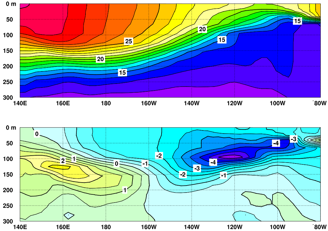
図3 2007年12月の太平洋の赤道に沿った水温(上)及び年間偏差(下)の断面図(海洋データ同化システムによる)。上図の等値線間隔は 1^{\circ}\text{C} 、下図の等値線間隔は 0.5^{\circ}\text{C} (年平均値は1987~2006年の20年平均値)。
