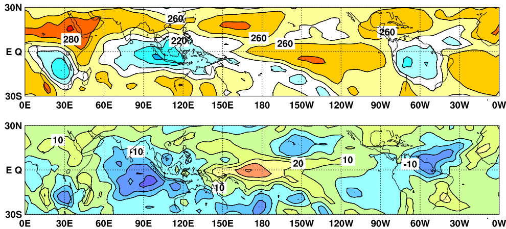
図 6 2007 年 12 月の外向き長波放射量 (OLR) ( 上 ) 及び平年偏差 ( 下 ) の分布図。OLR の値が小さいほど、対流活動が活発であることを示す。上図は 20\text{W/m}^2 毎、下図は 10\text{W/m}^2 毎に等値線を描いている ( 平年値は 1979 ~ 2004 年の 26 年平均値 )。OLR データは米国海洋大気庁 ( NOAA ) から提供されたものである。
