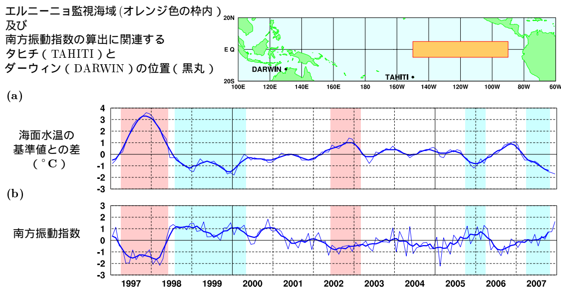
図1 エルニーニョ監視海域の海面水温の基準値との差( ^{\circ}\text{C} )(a)と南方振動指数(b)の推移(1997年1月~2007年12月)。折線は月平均値、滑らかな太線は5か月移動平均値を示す(海面水温の基準値はその年の前年までの30年間の各月の平均値、南方振動指数の平均値は1971~2000年の30年平均値)。赤色の陰影はエルニーニョ現象の発生期間を、青色の陰影はラニーニャ現象の発生期間を示している。
