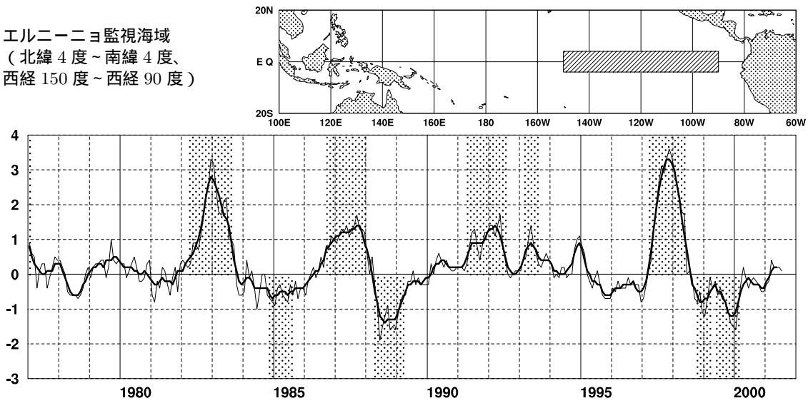
図 1 エルニーニョ監視海域の月平均海面水温の基準値との差 (°C) の推移 (1977 年 1 月 ~ 2001 年 7 月)。折線は月平均値、滑らかな太線は 5 か月移動平均値を示し、正の値は基準値より高いことを示す。エルニーニョ現象の発生期間は上側に、ラニーニャ現象の発生期間は下側に、それぞれ陰影を施してある (基準値は 1961 ~ 1990 年の 30 年平均値)。
