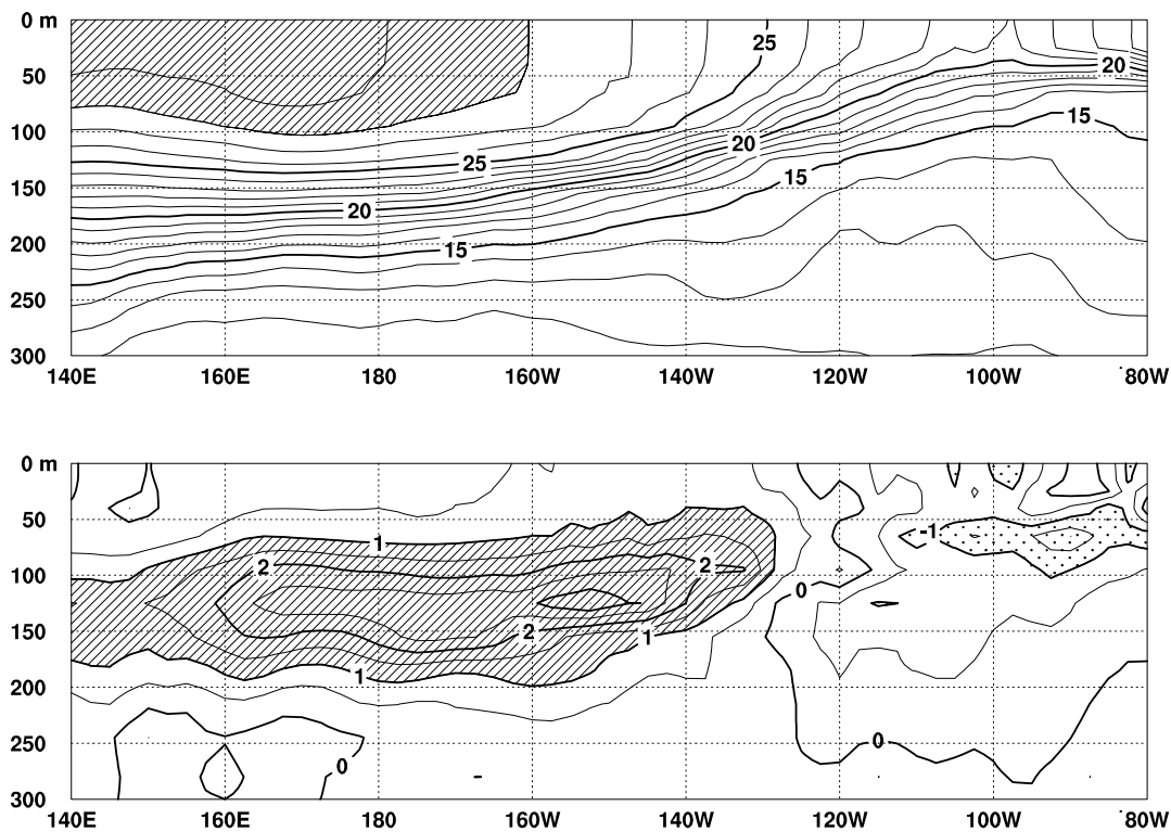
図3 2001年7月の太平洋の赤道に沿った水温(上)及び平年偏差(下)の断面図(海洋データ同化システムによる)。上図の等値線間隔は 1^{\circ}\text{C} で 28^{\circ}\text{C} 以上には陰影を施し、下図の等値線間隔は 0.5^{\circ}\text{C} で +1^{\circ}\text{C} 以上( -1^{\circ}\text{C} 以下)の偏差には濃い(薄い)陰影を施した(平年値は1987~1999年の13年平均値)。
