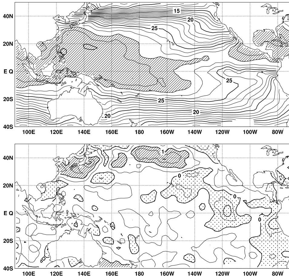
図 2 2001 年 7 月の海面水温図 (上) 及び平年偏差図 (下)。海面水温図の大線は 5°C 毎、細線は 1°C 毎の、平年偏差図の大線は 1°C 毎、細線は 0.5°C 毎の等値線を示す。海面水温図の陰影部は 28°C 以上の領域を、偏差図の濃い (薄い) 陰影部は +1°C 以上の正偏差域 (0°C 以下の負偏差域) を示す (平年値は 1971 ~ 2000 年の 30 年平均値)。
