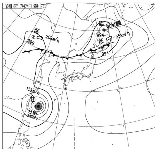
7 月 24 日 09 時の地上天気図（左）と気象衛星赤外画像（右）
