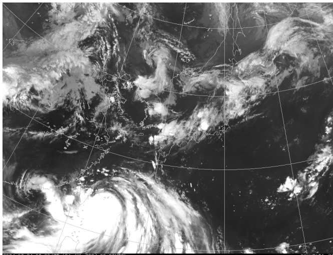
7 月 24 日 09 時の地上天気図（左）と気象衛星赤外画像（右）
