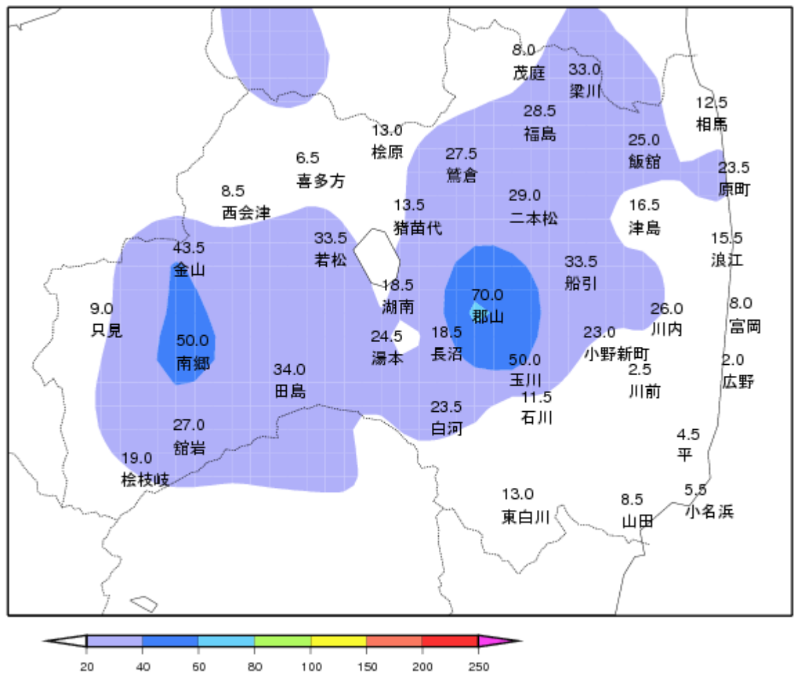
資料 3 アメダス降水量分布図(6 日 12 時～7 日 06 時の合計)
