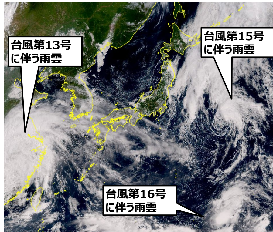
10日11時30分の気象衛星画像（可視画像）
