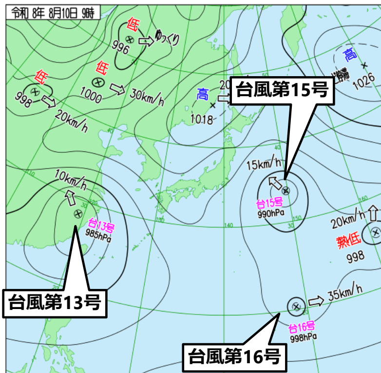
10日9時の実況天気図
