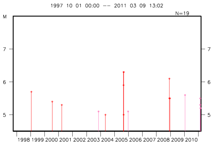
震央分布図領域a内の地震活動経過図 (1997年10月1日～、深さ200km以浅、 M5.0以上)
