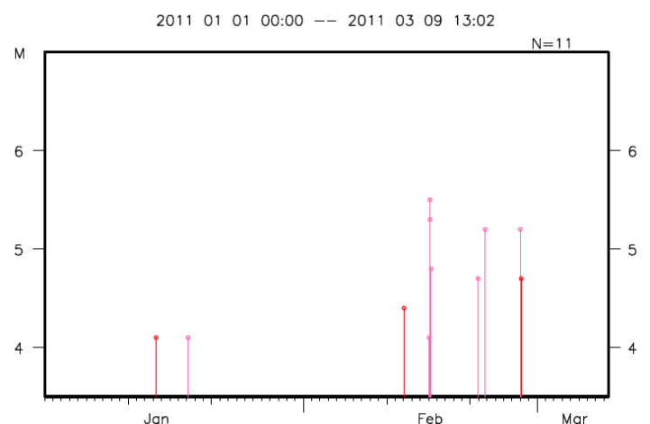
震央分布図領域a内の地震活動経過図 (2011年1月1日～、深さ200km以浅、 M4.0以上)
