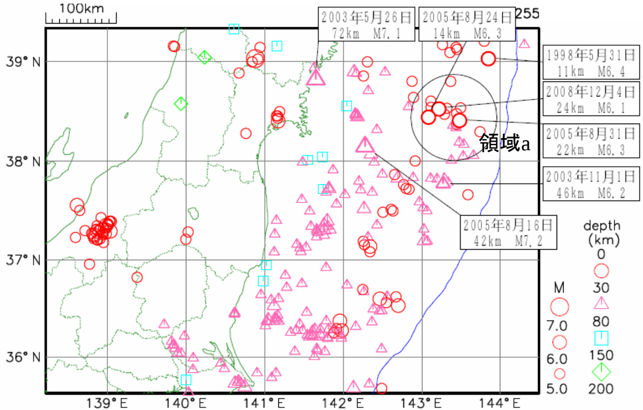
震央分布図(1997年10月1日～、深さ200km以浅、M5.0以上)
