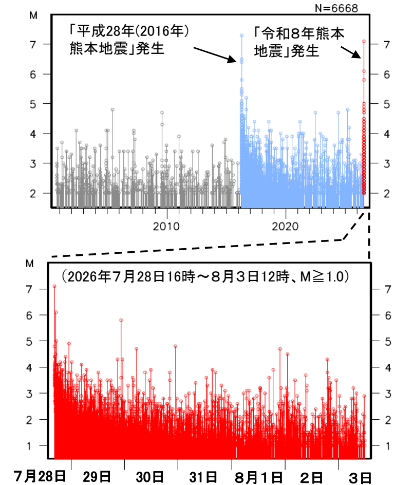
領域a内の地震活動経過図
