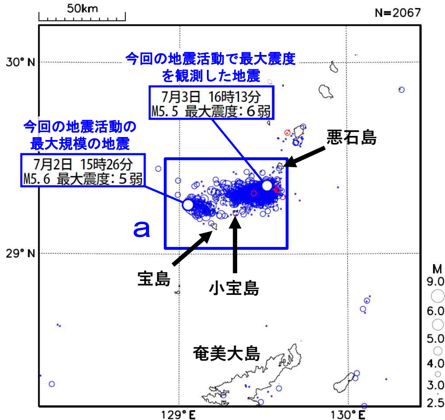
震央分布図
