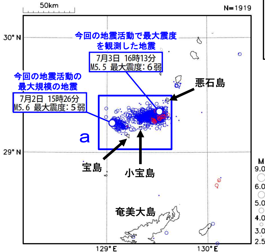
震央分布図
