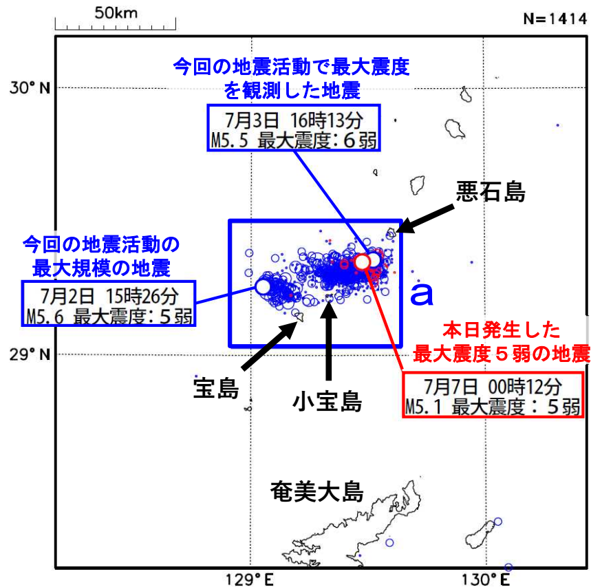
震央分布図
