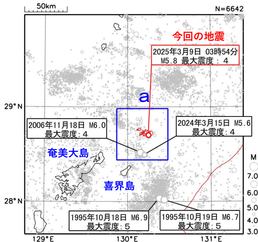
震央分布図
