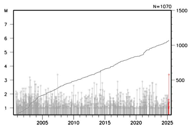
図7 図6領域a内の地震活動経過図 及び回数積算図
