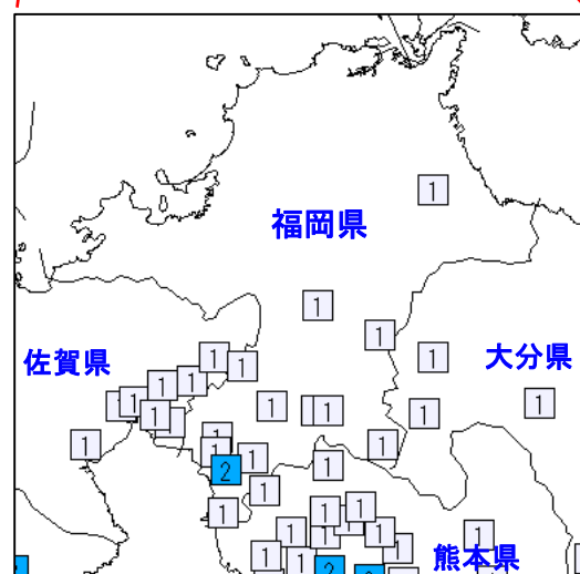
図 1 震度分布図 （上段：地域別、下段：観測点別） 18 日 05 時 00 分 M4.8
