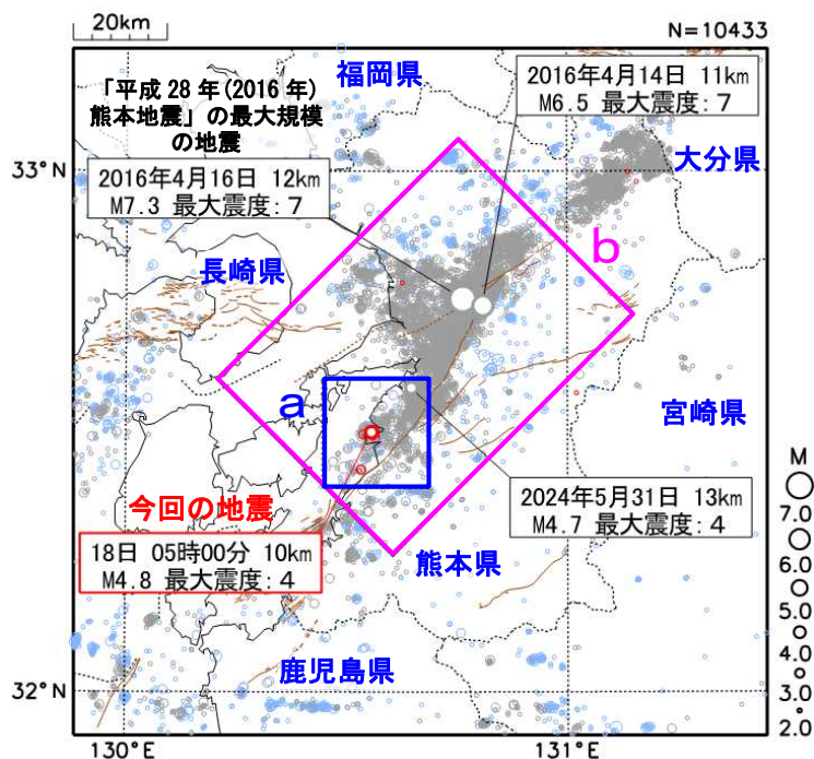
図 2 震央分布図 （2000 年 10 月 1 日～2025 年 3 月 31 日、 深さ 0～20km、M≥2.0）
