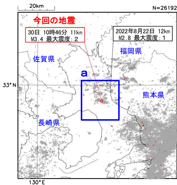
図6 震央分布図 (2000年10月1日～2025年3月31日、 深さ0～20km、 M \geq 1.0 ) ※ 2025年3月の地震を赤色○で表示
