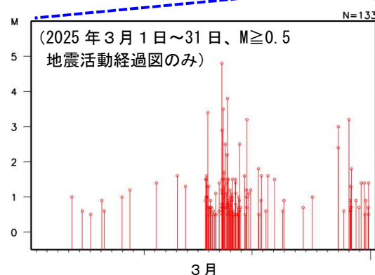
図 3 図 2 領域 a 内の地震活動経過図 及び回数積算図
