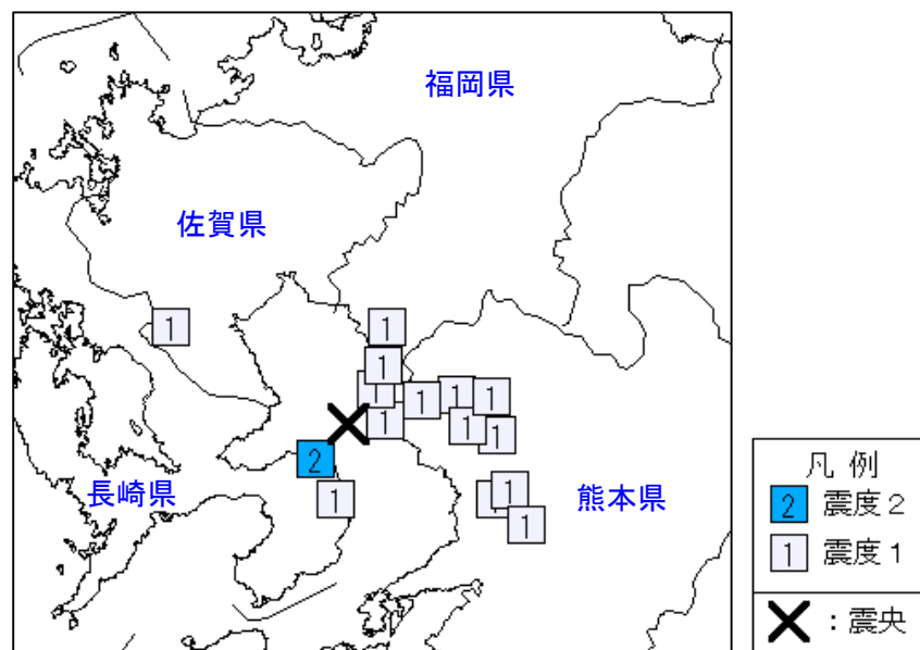
図5 震度分布図（観測点別） 30日10時46分 M3.4
