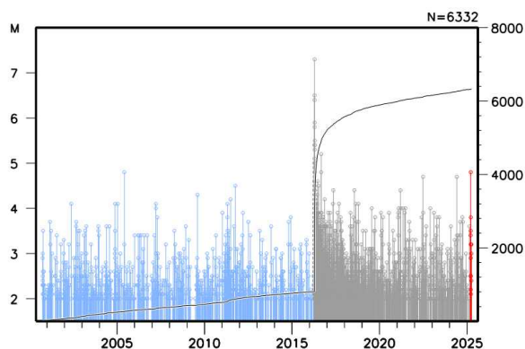
図 4 図 2 領域 b 内の地震活動経過図 及び回数積算図
