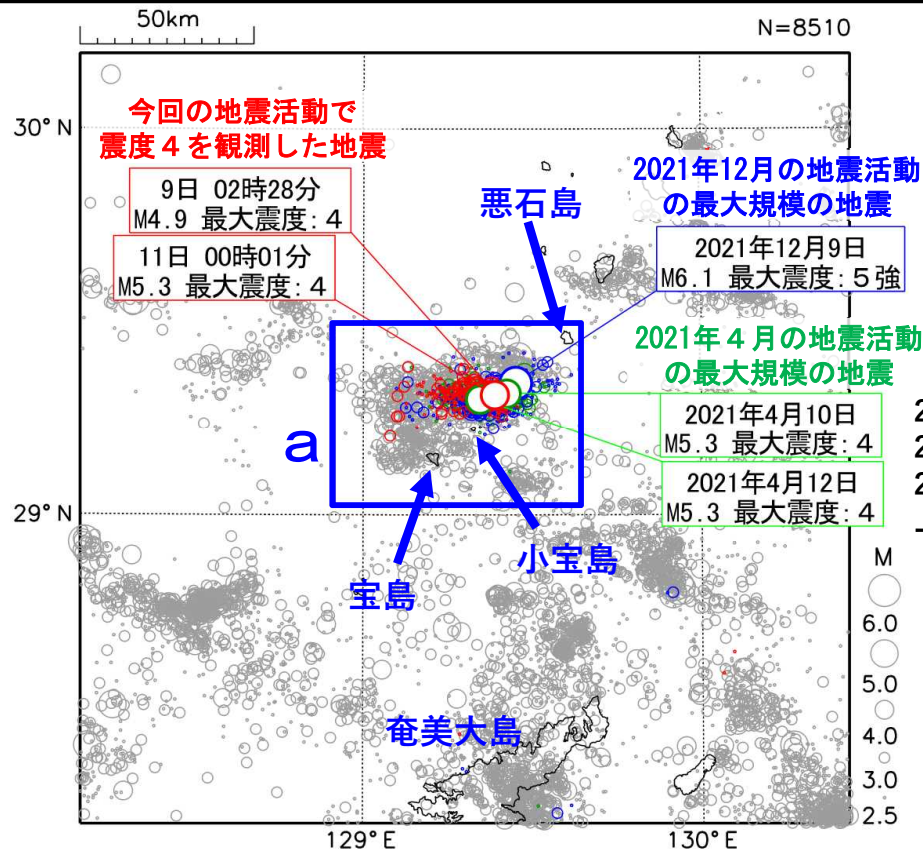
震央分布図
