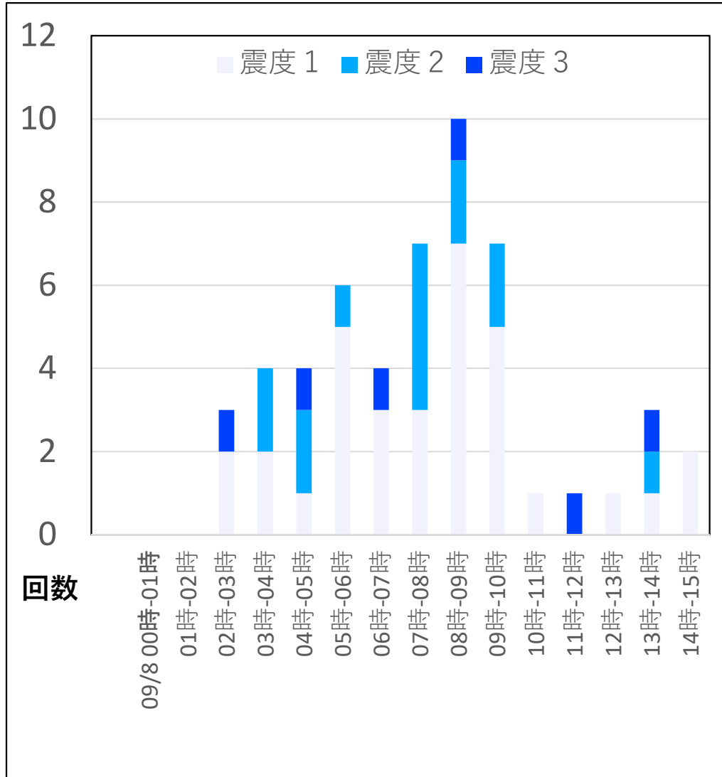
【時別地震回数図】
