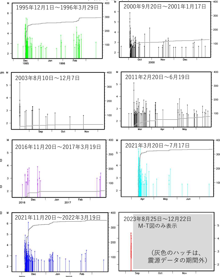
領域a内の期間別（各120日間）の地震活動経過図及び 回数積算図
