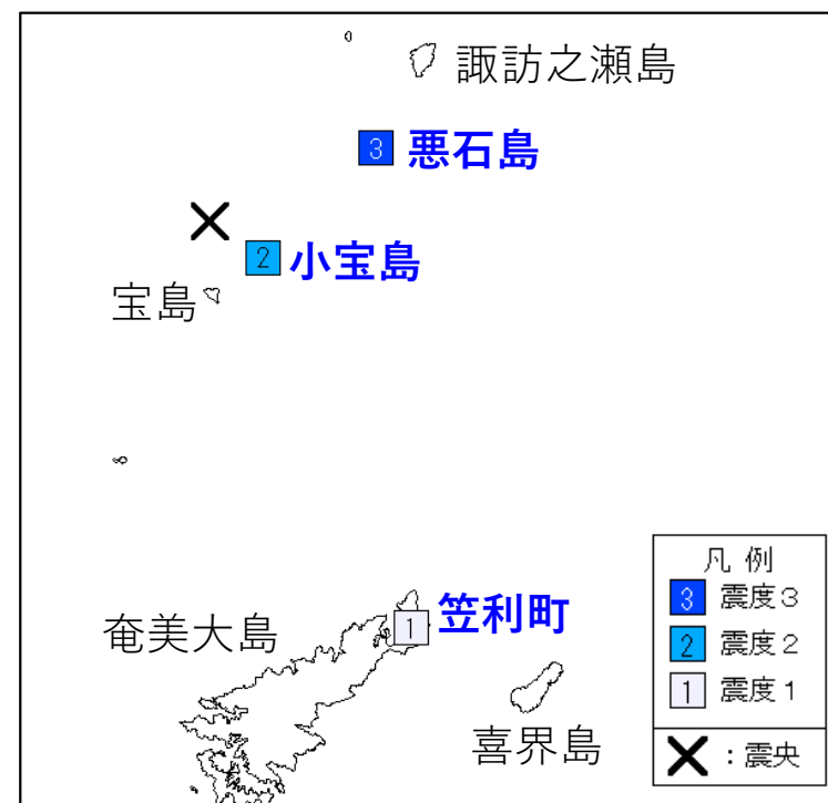
本日の最大規模の地震の震度分布図 8日13時15分頃 M4.6（速報値）
