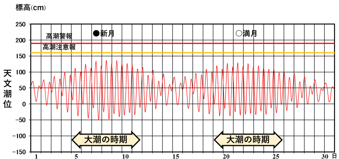
図3 博多における2021年9月（1時間ごとの）の天文潮位
