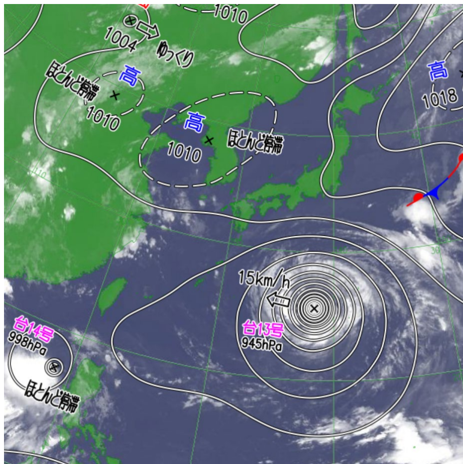
気象衛星画像と天気図(5日9時)
